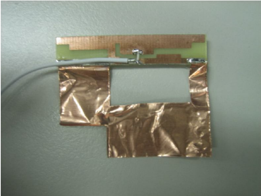
(14) EUT Photo (YAGEO Antenna-Aux)
