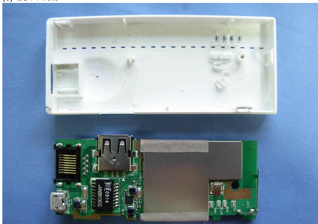
(9) EUT Photo
