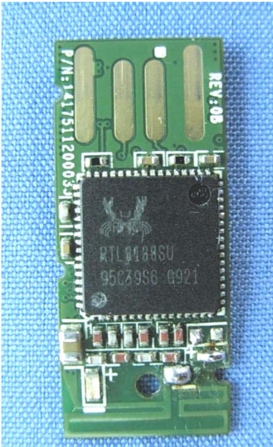
(13) EUT Photo
