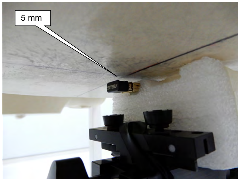
EUT Back
