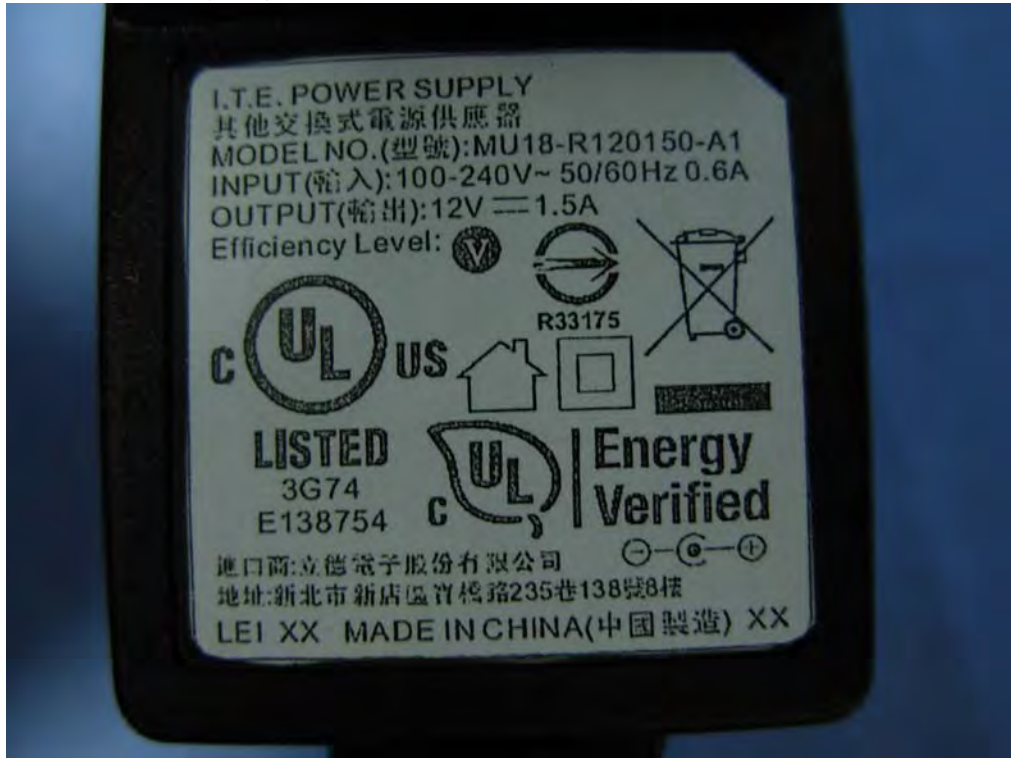
(120) EUT Photo(Adapter:ITE,MU18-R120150-A1)
