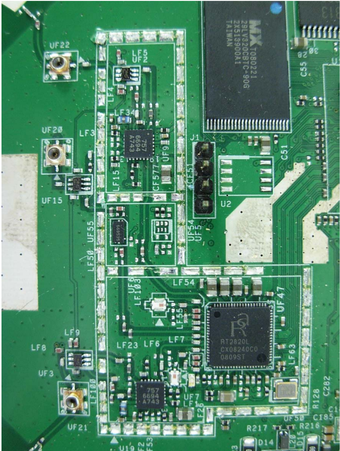
(9) EUT Photo
