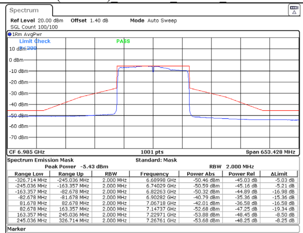
802.11ax (160MHz) 6985MHz Chain D NSS-1
