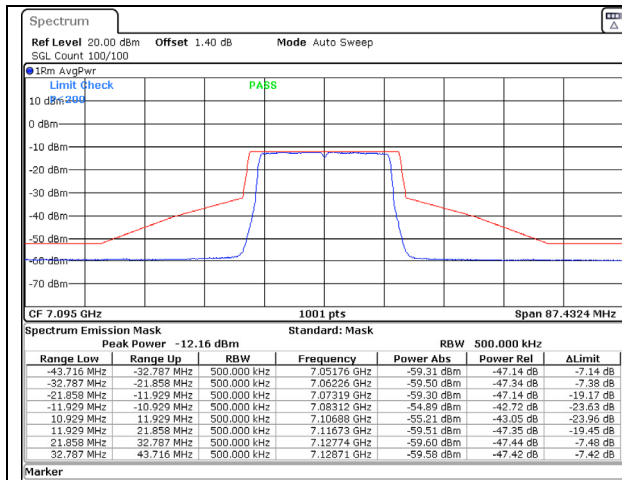
802.11ax (20MHz) 7095MHz Chain A NSS-2
