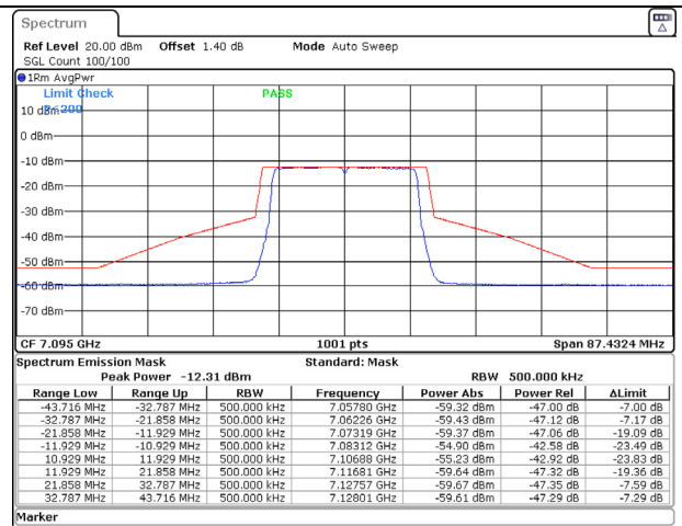
802.11ax (20MHz) 7095MHz Chain B NSS-2
