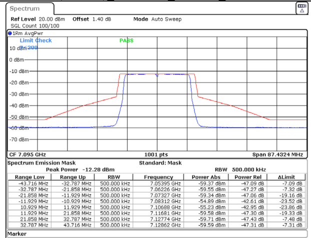
802.11ax (20MHz) 7095MHz Chain D NSS-2
