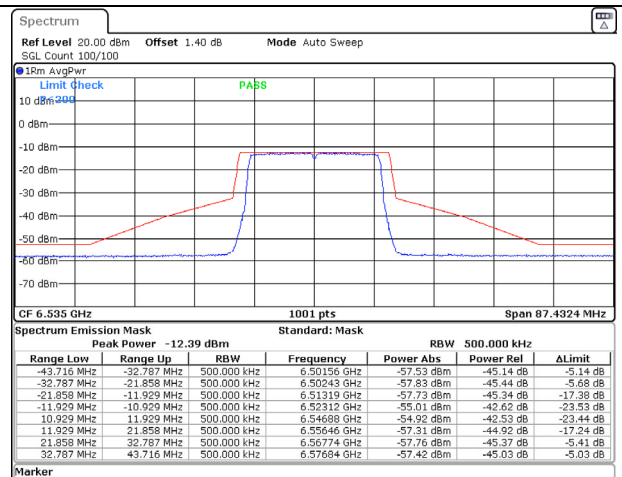
802.11ax (20MHz) 6535MHz Chain B NSS-2
