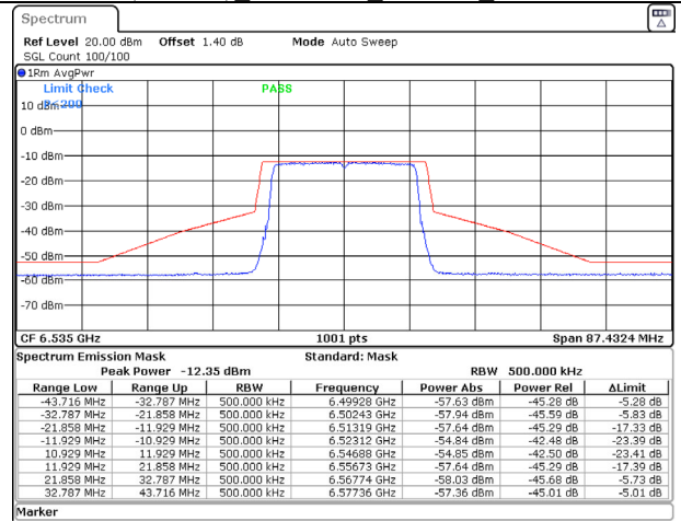
802.11ax (20MHz) 6535MHz Chain D NSS-2
