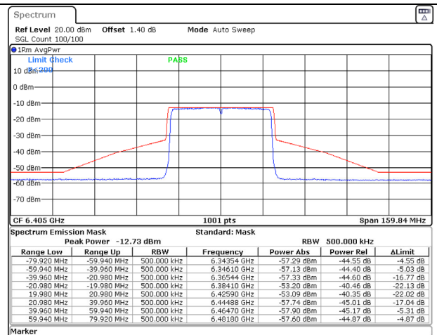
802.11ax (40MHz) 6405MHz Chain B NSS-2
