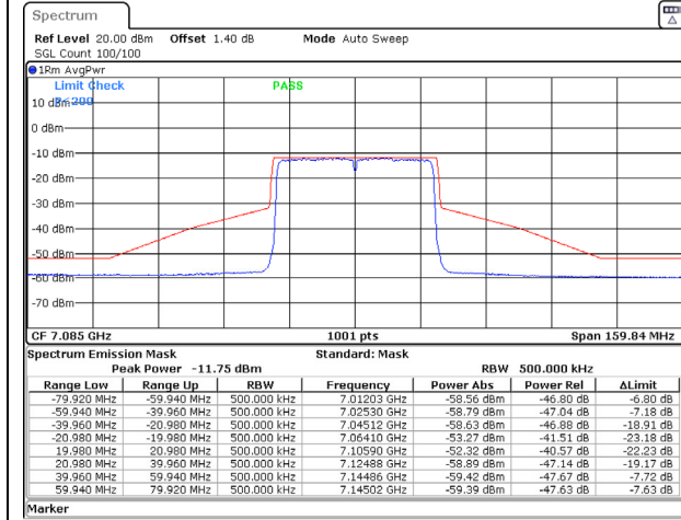
802.11ax (40MHz) 7085MHz Chain A NSS-2
