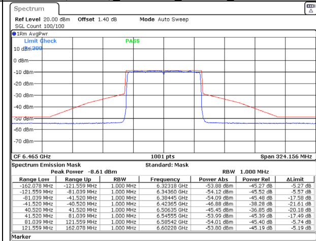
802.11ax (80MHz) 6465MHz Chain B NSS-2
