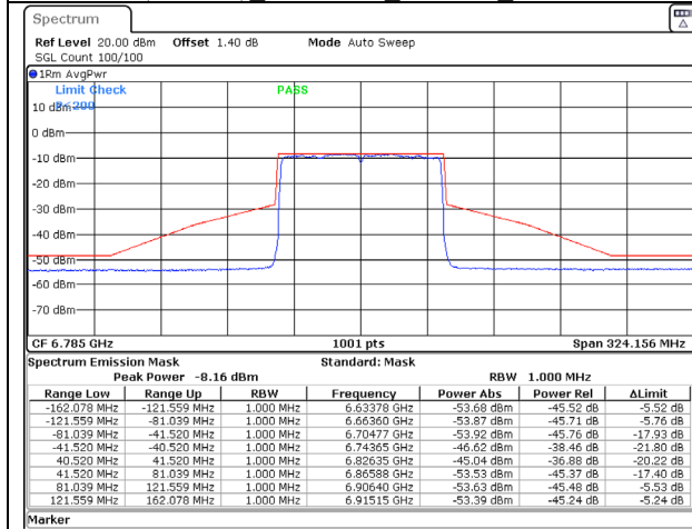
802.11ax (80MHz) 6785MHz Chain C NSS-2
