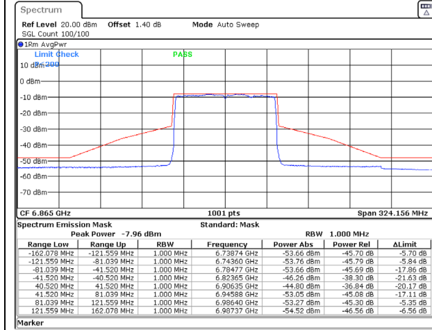
802.11ax (80MHz) 6865MHz Chain A NSS-2
