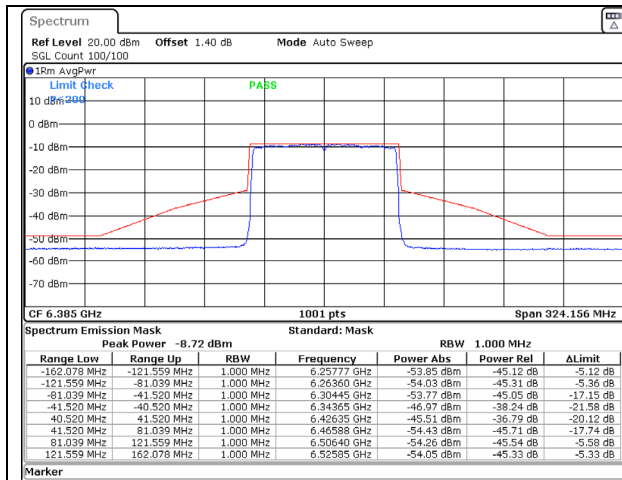
802.11ax (80MHz) 6385MHz Chain C NSS-2
