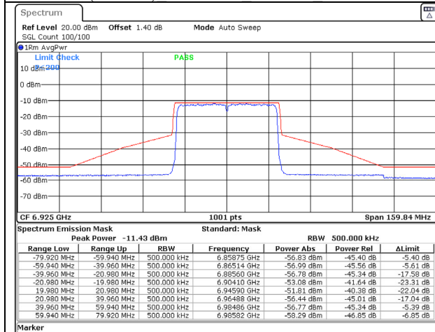
802.11ax (40MHz) 6925MHz Chain C NSS-2
