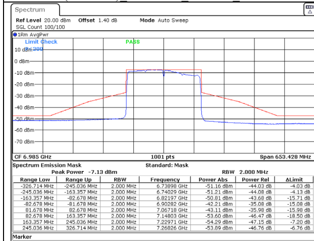
802.11ax (160MHz) 6985MHz Chain C NSS-2
