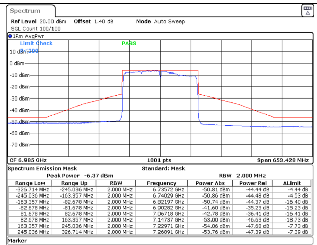
802.11ax (160MHz) 6985MHz Chain B NSS-2
