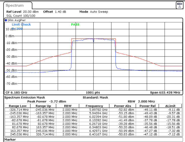
802.11ax (160MHz) 6185MHz Chain D NSS-2
