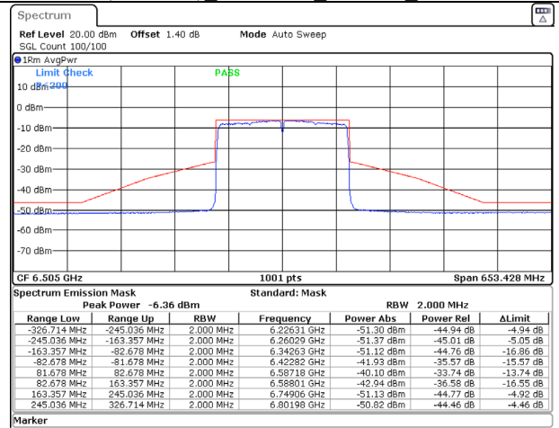
802.11ax (160MHz) 6505MHz Chain D NSS-2
