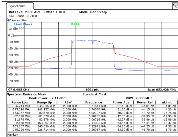
802.11ax (160MHz) 6985MHz Chain A NSS-2
