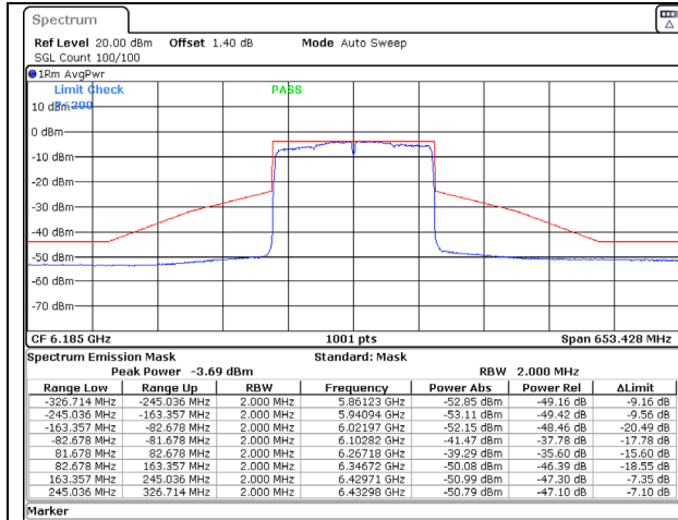
802.11ax (160MHz) 6185MHz Chain C NSS-2
