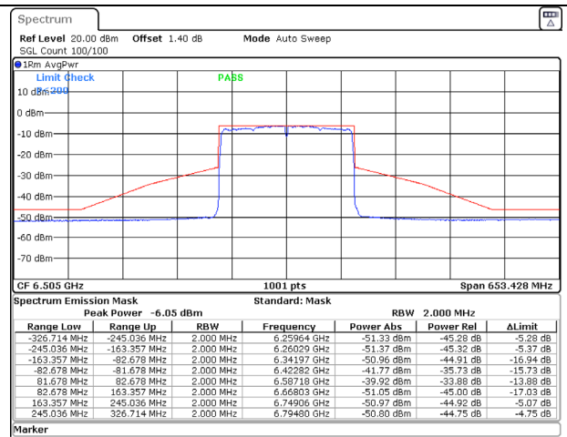
802.11ax (160MHz) 6505MHz Chain B NSS-2
