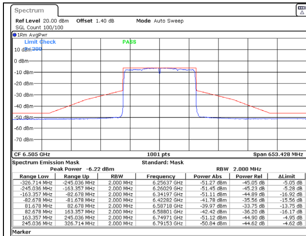
802.11ax (160MHz) 6505MHz Chain A NSS-2
