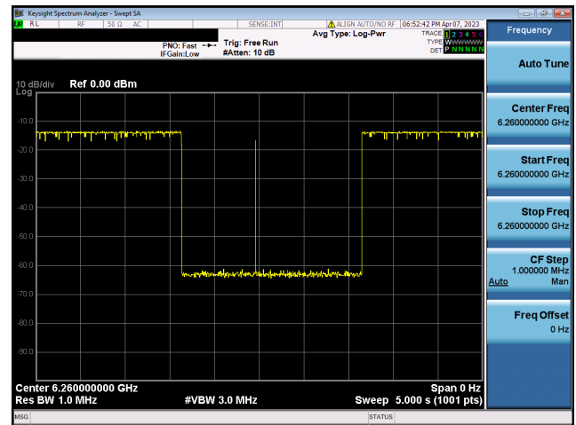
802.11ax (160MHz) / 6260MHz (High Edge - 6260MHz)
