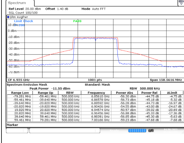
802.11ax (40MHz) 6925MHz Chain D NSS-1
