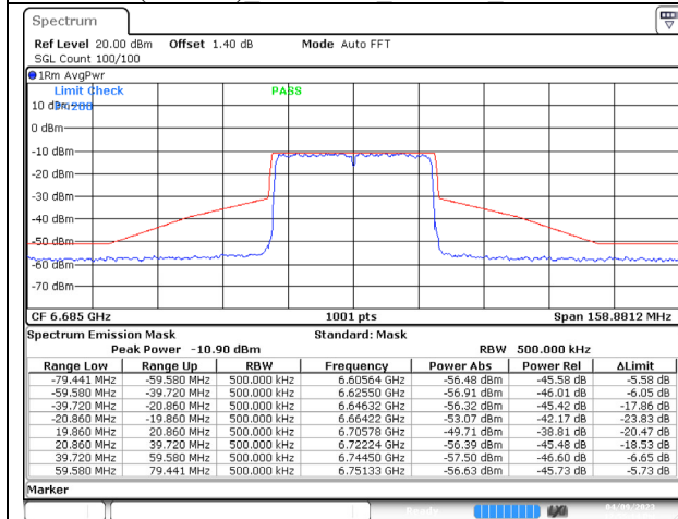
802.11ax (40MHz) 6685MHz Chain A NSS-4
