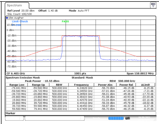
802.11ax (40MHz) 6405MHz Chain B NSS-4
