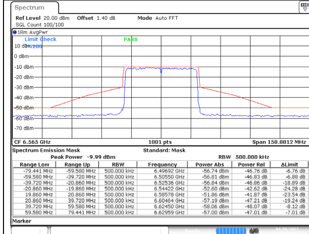
802.11ax (40MHz) 6565MHz Chain A NSS-4
