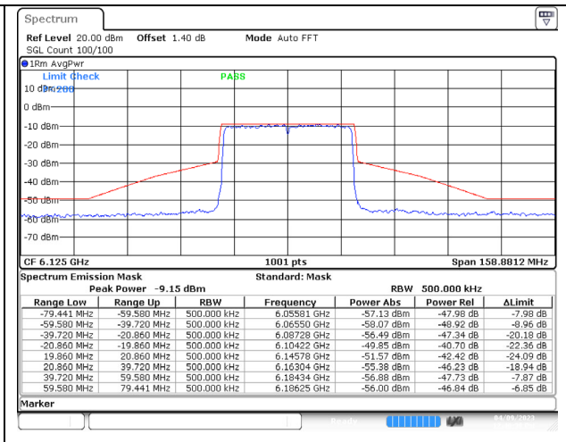
802.11ax (40MHz) 6125MHz Chain D NSS-4
