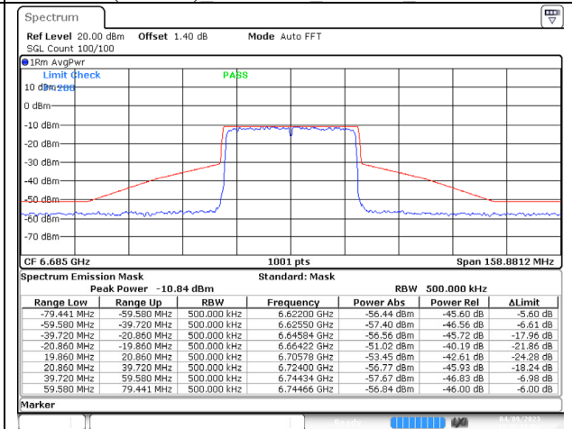
802.11ax (40MHz) 6685MHz Chain B NSS-4
