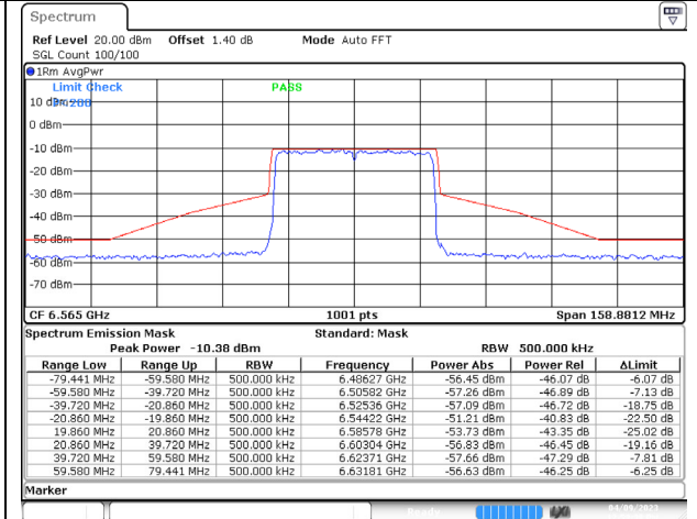
802.11ax (40MHz) 6565MHz Chain B NSS-4
