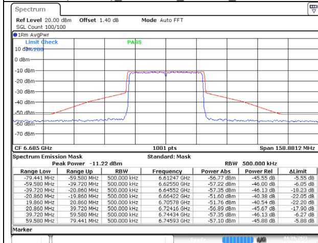
802.11ax (40MHz) 6685MHz Chain C NSS-4
