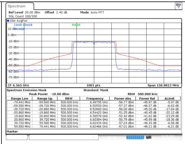
802.11ax (40MHz) 6565MHz Chain D NSS-4
