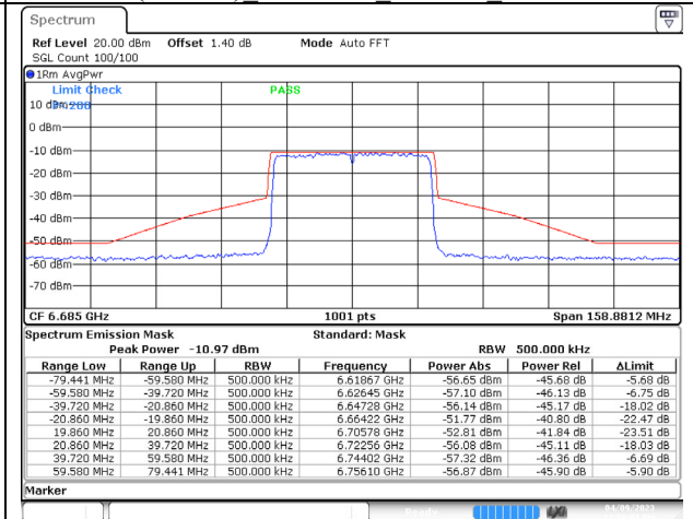
802.11ax (40MHz) 6685MHz Chain D NSS-4
