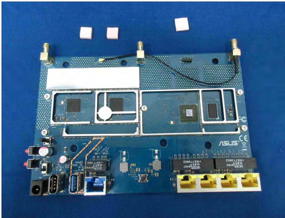
(20) EUT Photo
