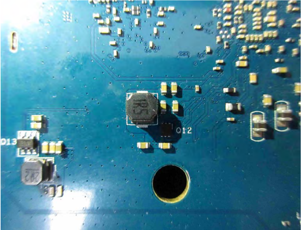
(8) EUT Photo
