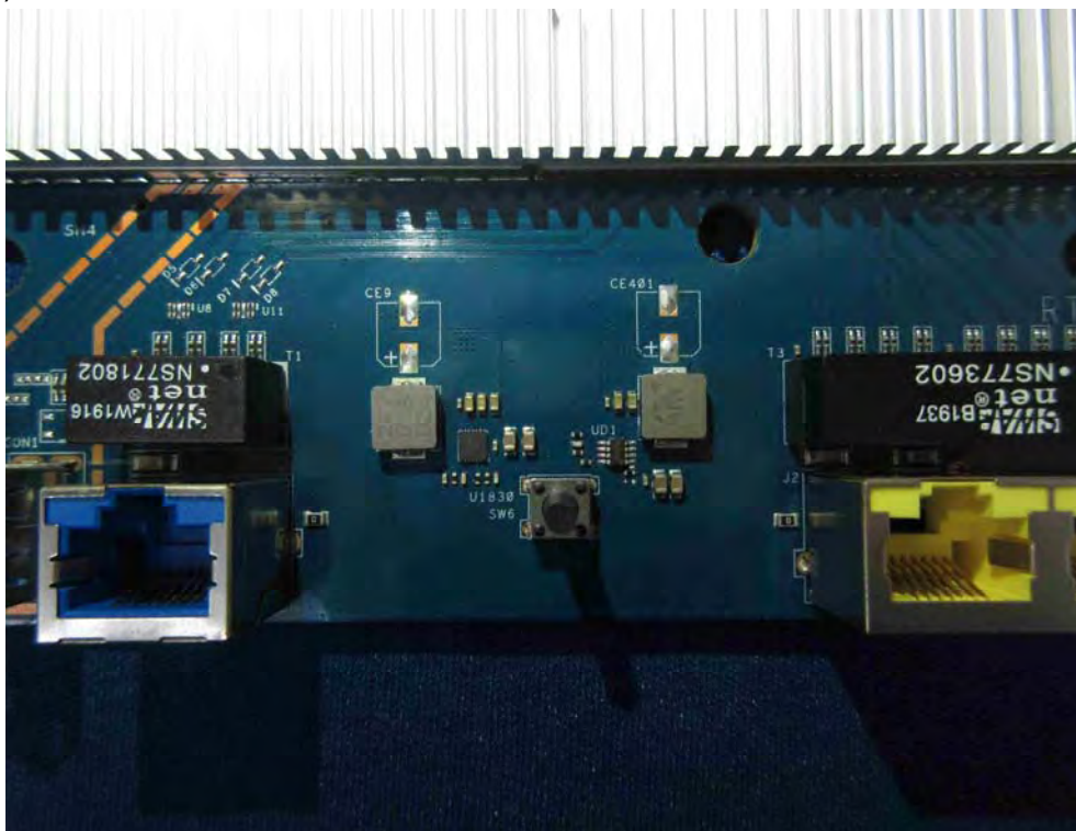
(16) EUT Photo
