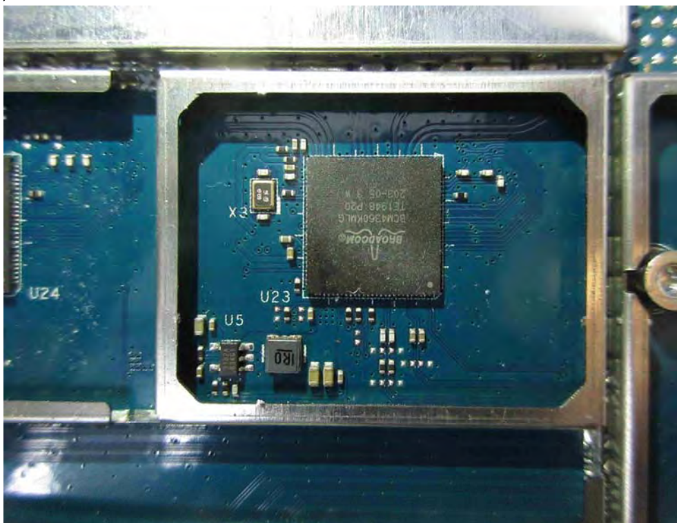
(30) EUT Photo
