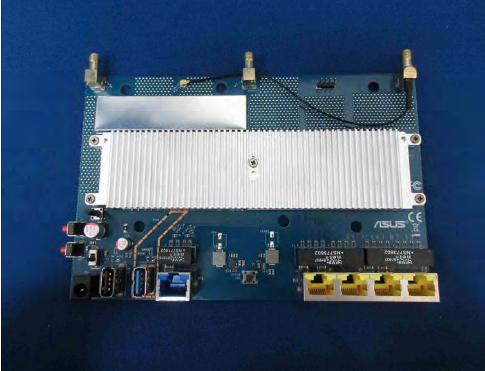
(4) EUT Photo
