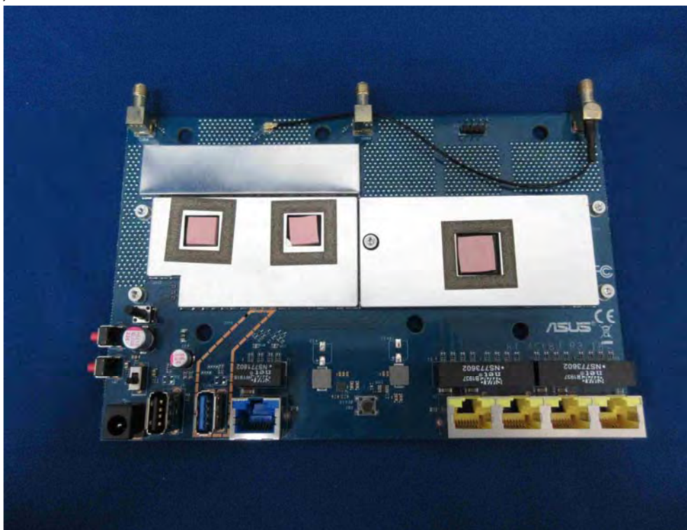
(18) EUT Photo
