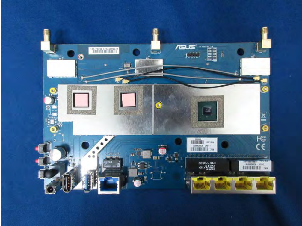
(64) EUT Photo
