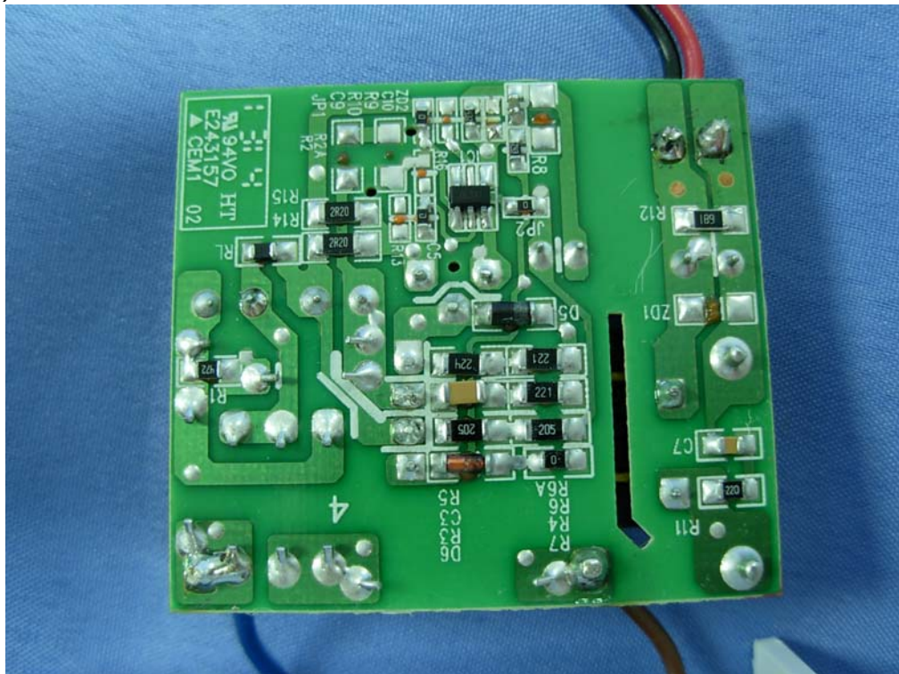
(37) EUT Photo
