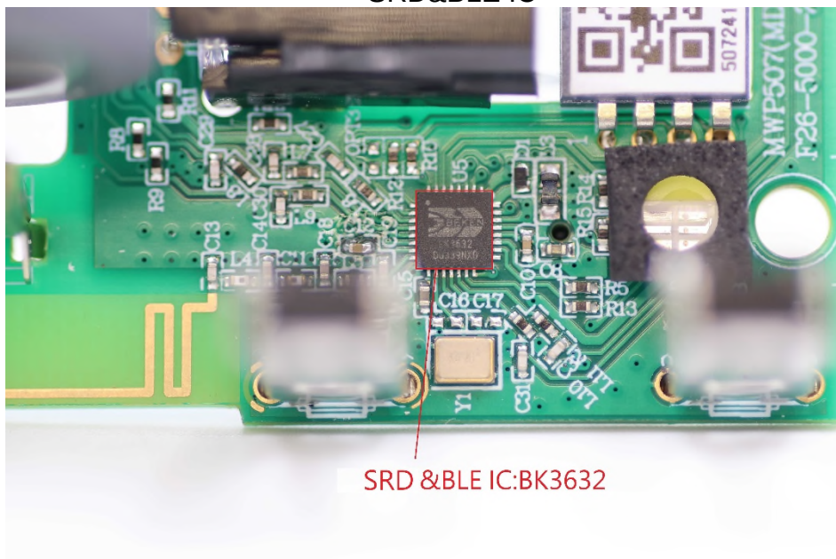
SRD&amp;BLE IC
