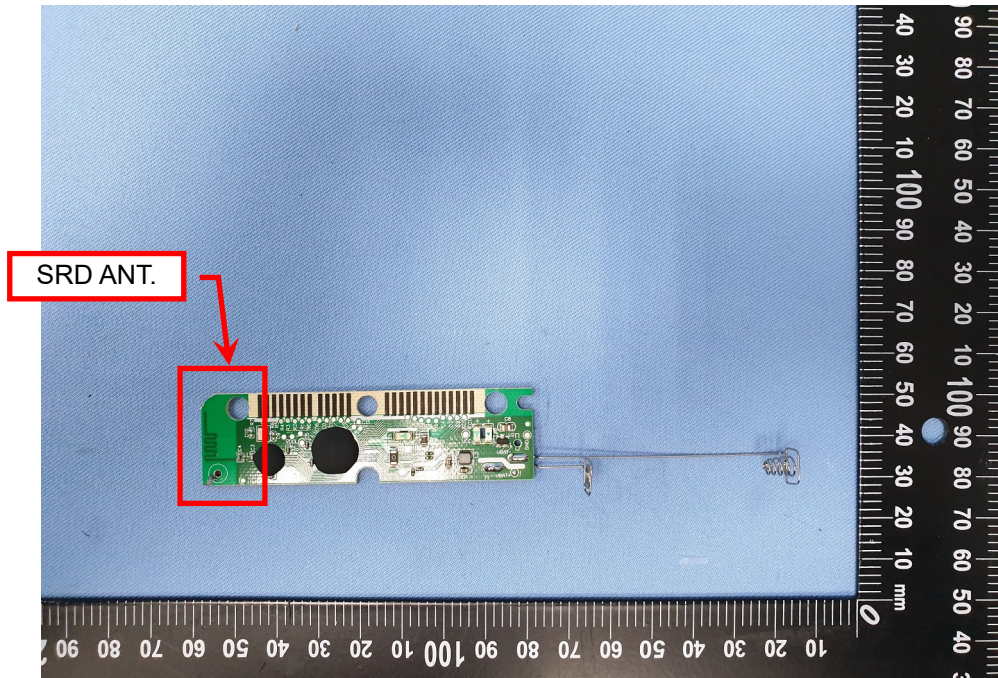
EUT Photo (6)
