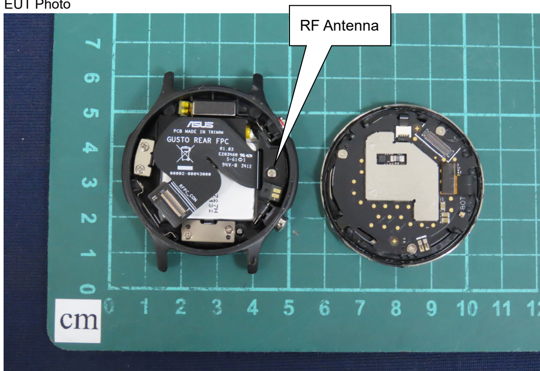
(9) EUT Photo
