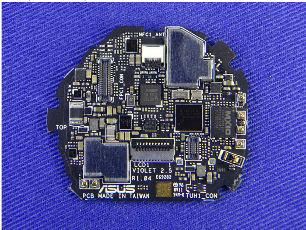
(24) EUT Photo (M/N: HC-A05)
