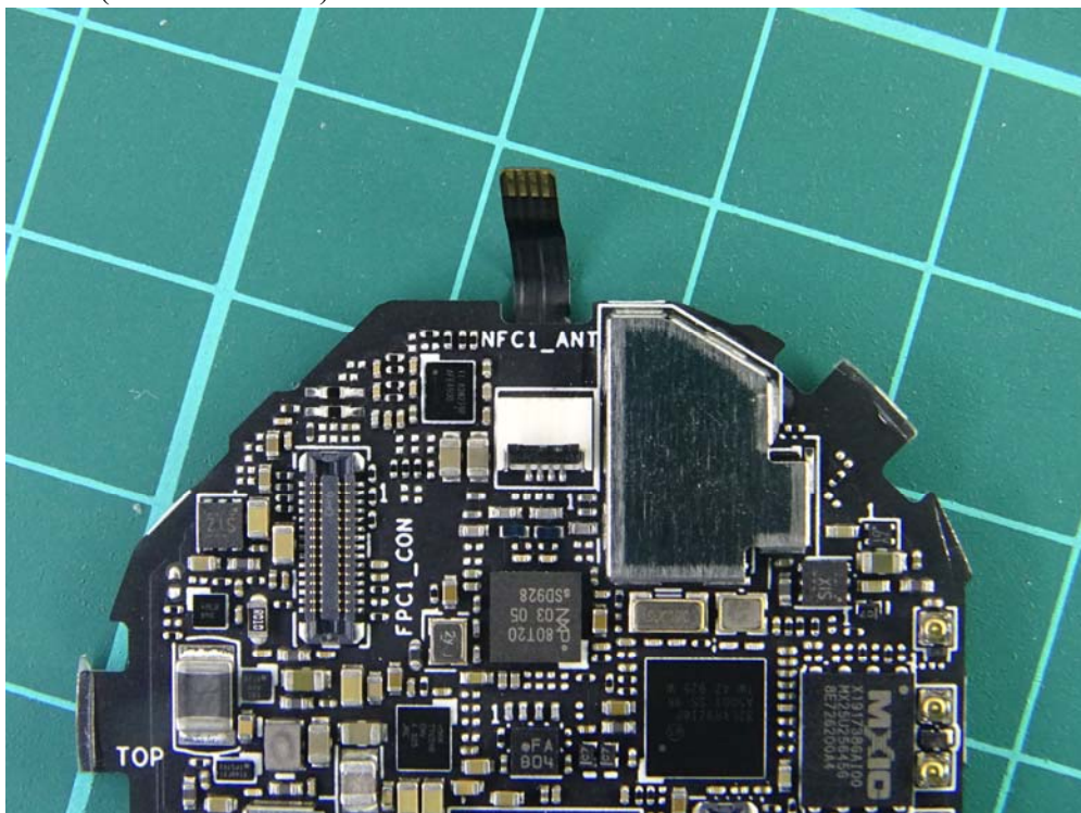
(60) EUT Photo (M/N: HC-A05K)
