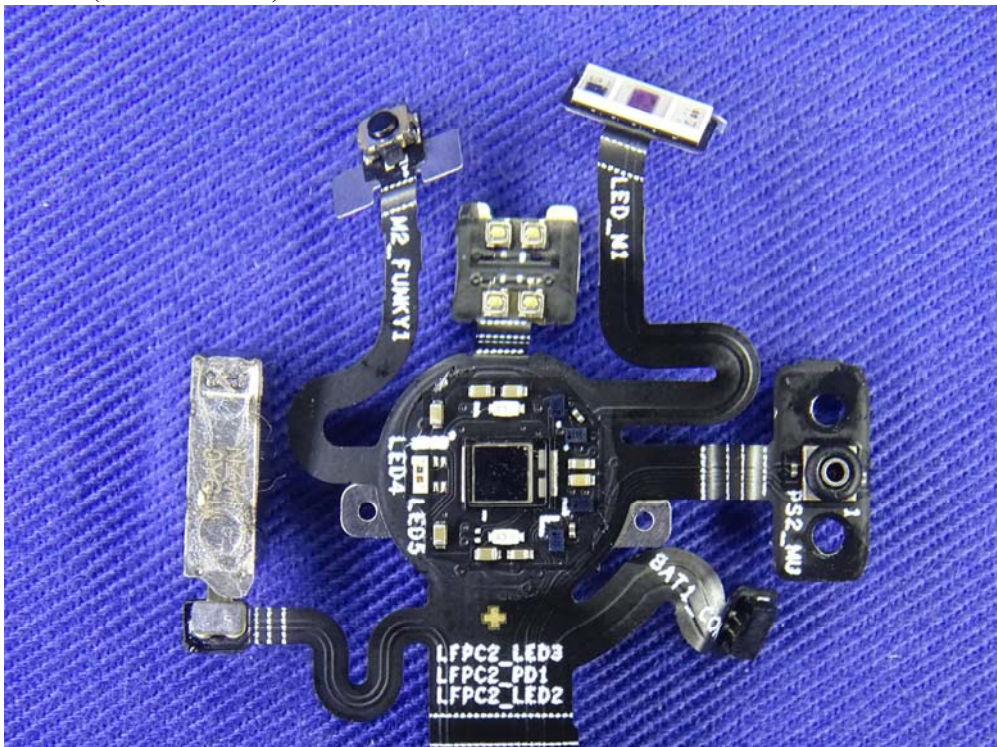
(10) EUT Photo (M/N: HC-A05)
