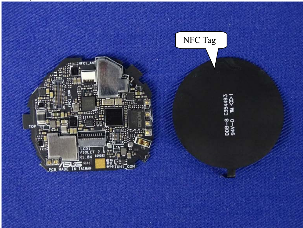
(23) EUT Photo (M/N: HC-A05)
