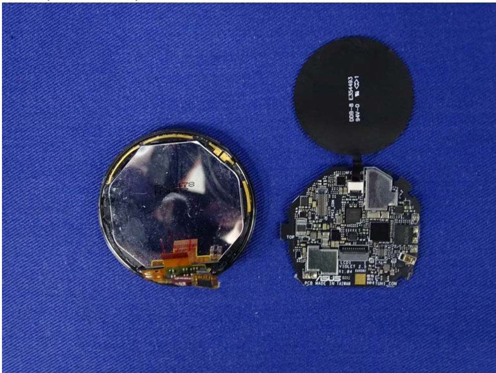
(18) EUT Photo (M/N: HC-A05)
