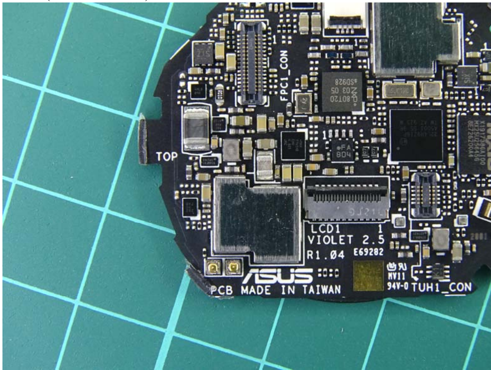
(61) EUT Photo (M/N: HC-A05K)
