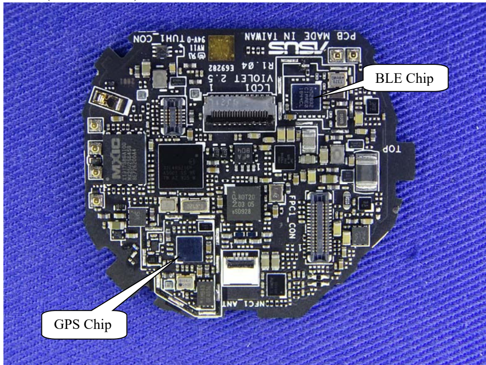
(25) EUT Photo (M/N: HC-A05)
