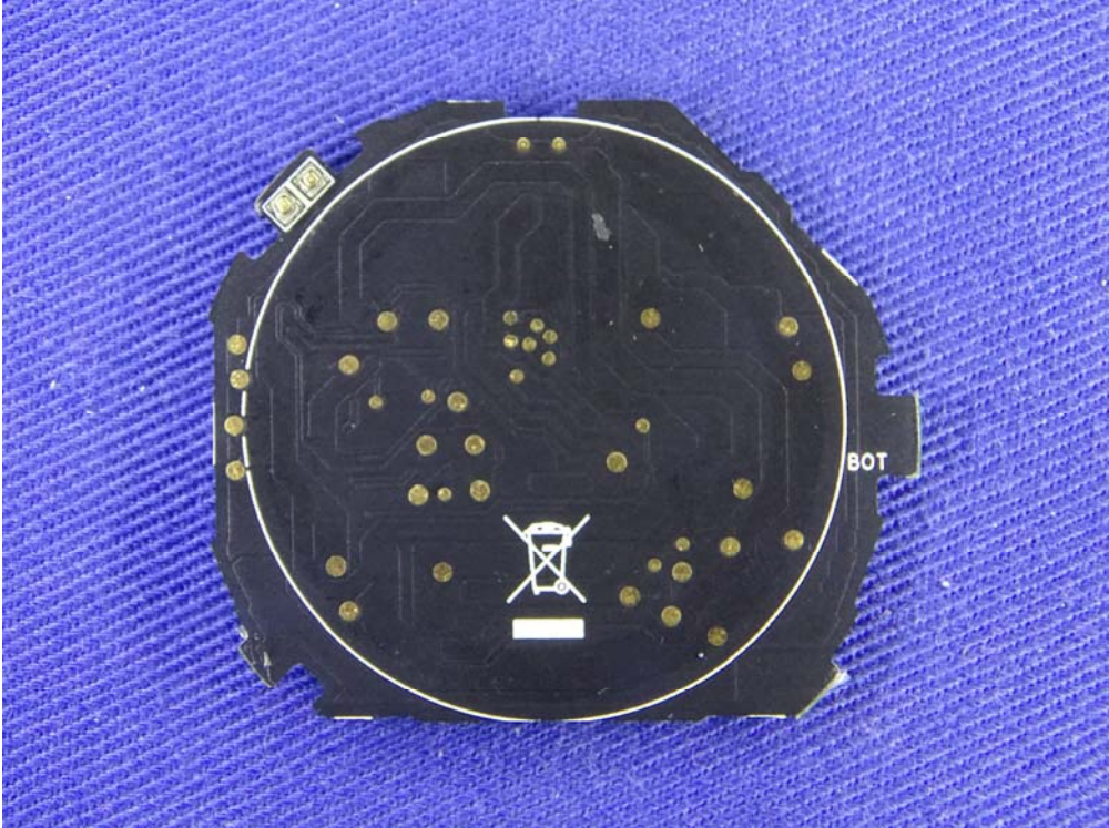
(29) EUT Photo (M/N: HC-A05)
