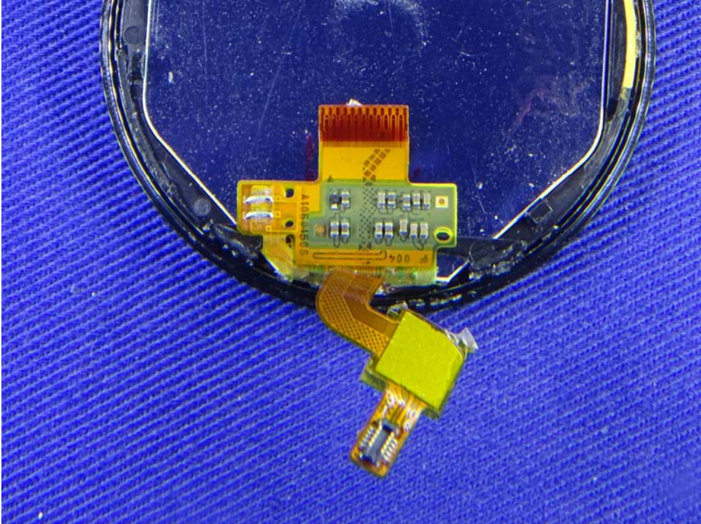
(21) EUT Photo (M/N: HC-A05)
