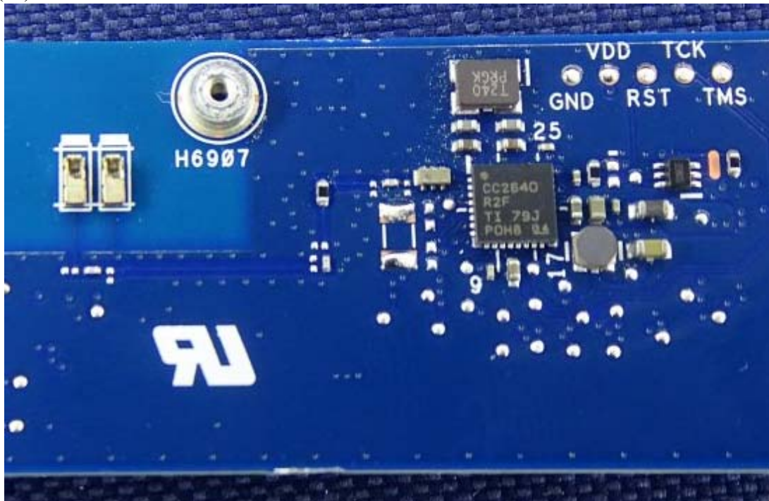
(33) EUT Photo
