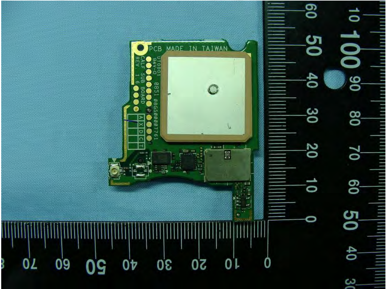
GPS Antenna
