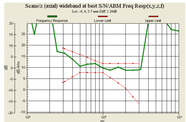
Fig. 9.6 GSM1900 Ch810
