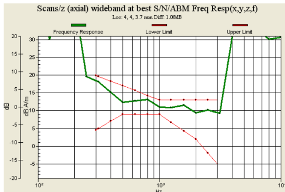
Fig. 9.3 GSM850 Ch251
