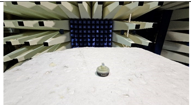
Fig A6: EUT Close up
