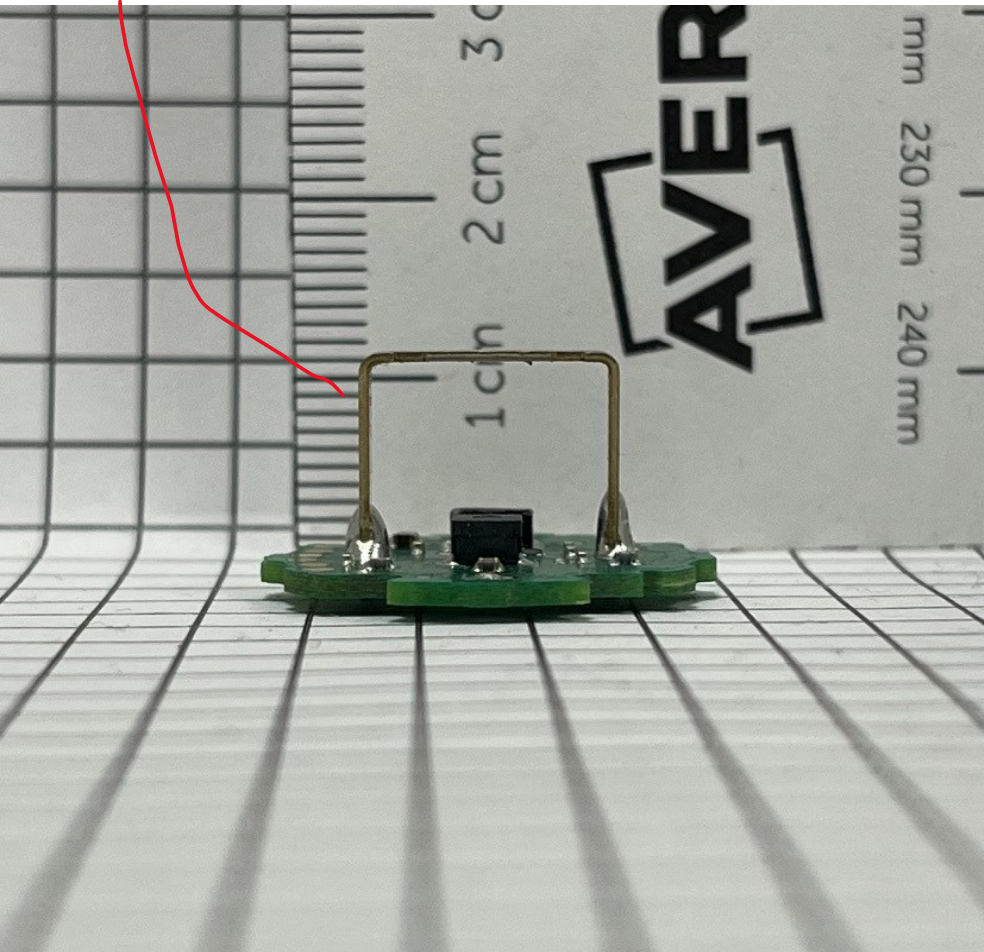
Antenna
