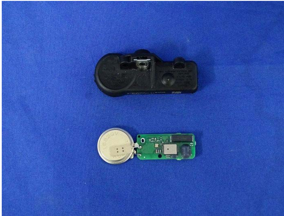
(5) EUT Photo
