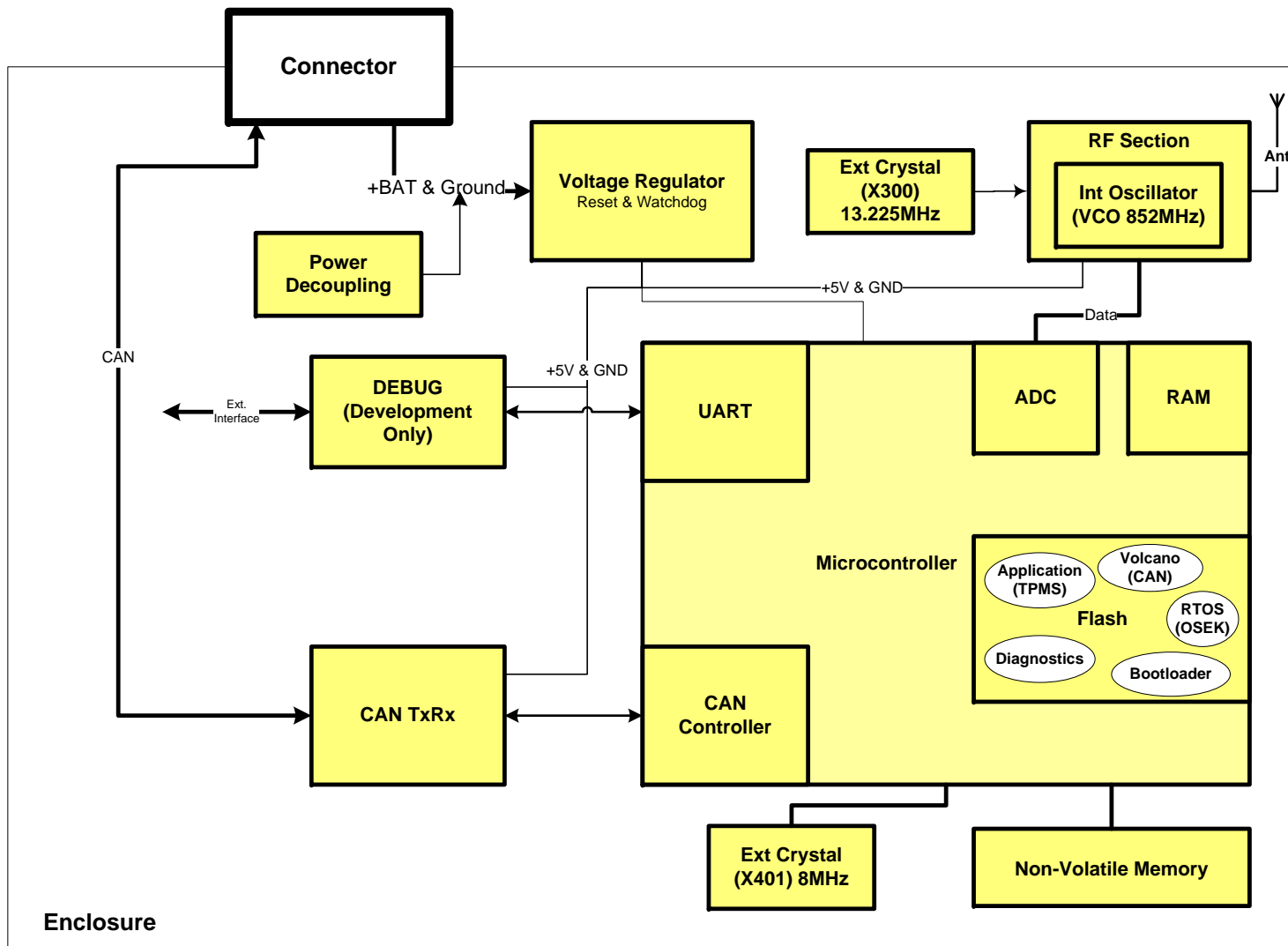
Fig. 2 : Mercedes Corax Block Diagram
