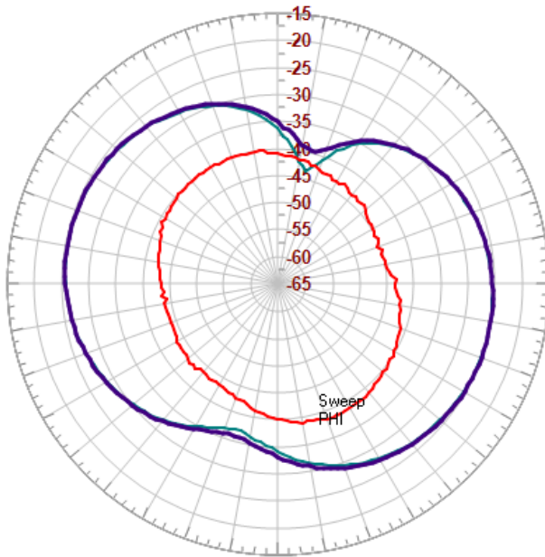
Theta = 90 (dBi)
