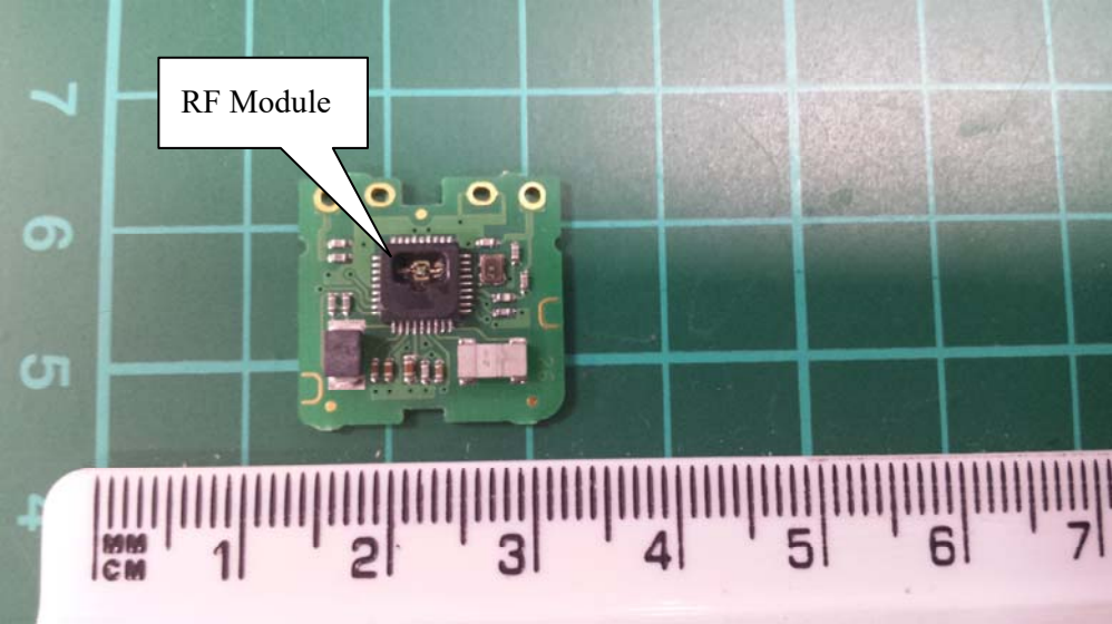
(8) EUT Photo
