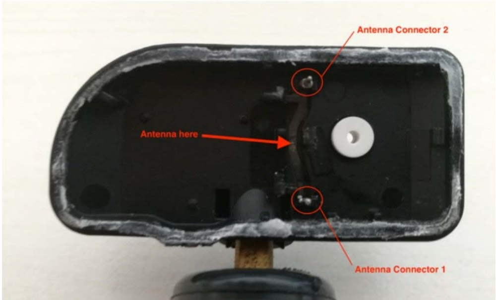
(10) EUT Photo
