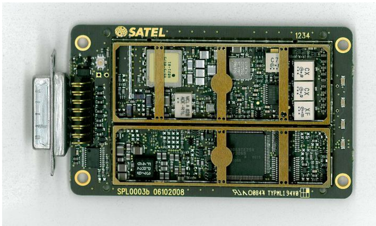
SATEL-TA10 frontside
