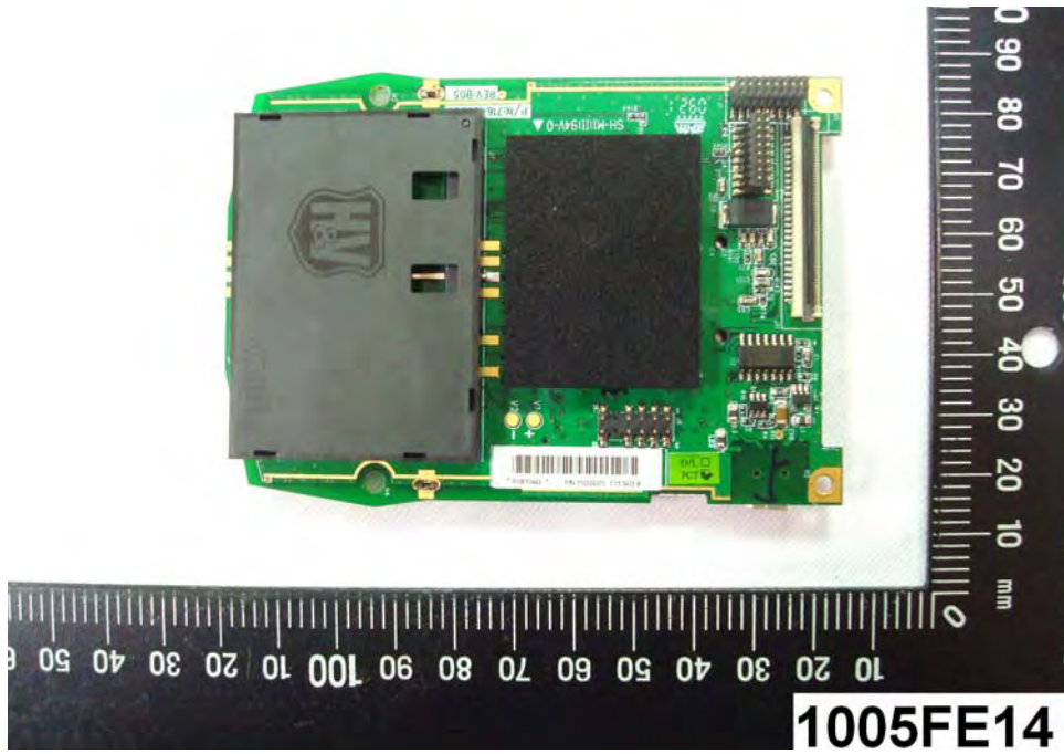
(17) EUT Photo
