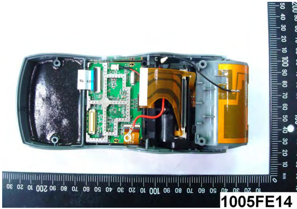
(21) EUT Photo
