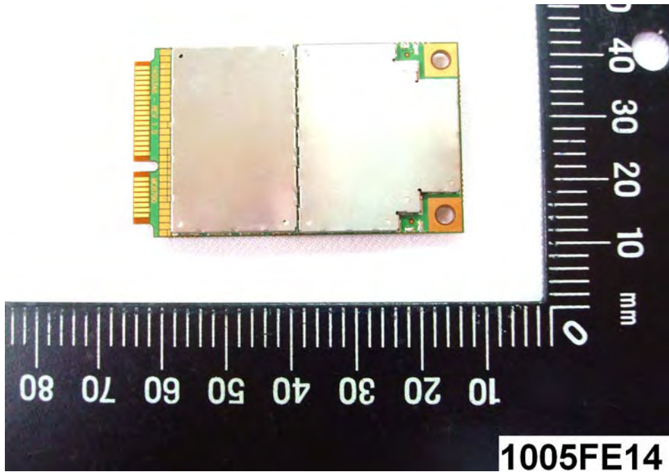
(9) EUT Photo
