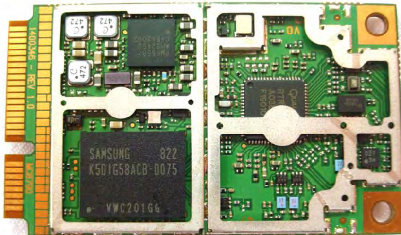
(10) EUT Photo
