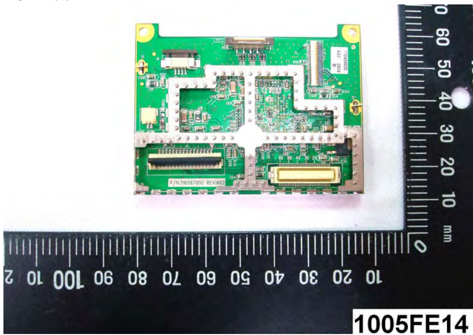
(24) EUT Photo
