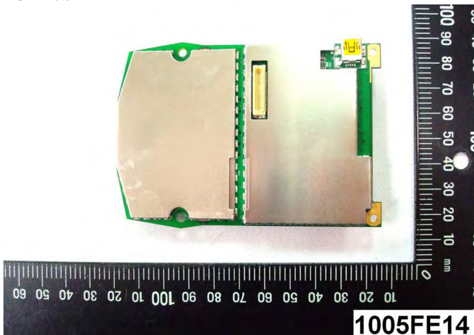
(18) EUT Photo
