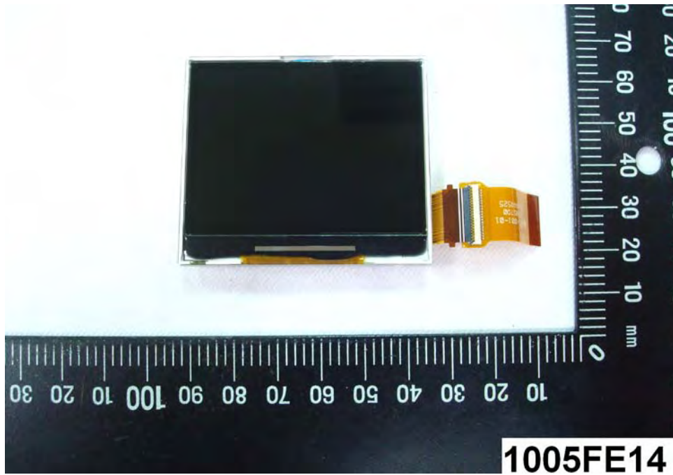
(30) EUT Photo
