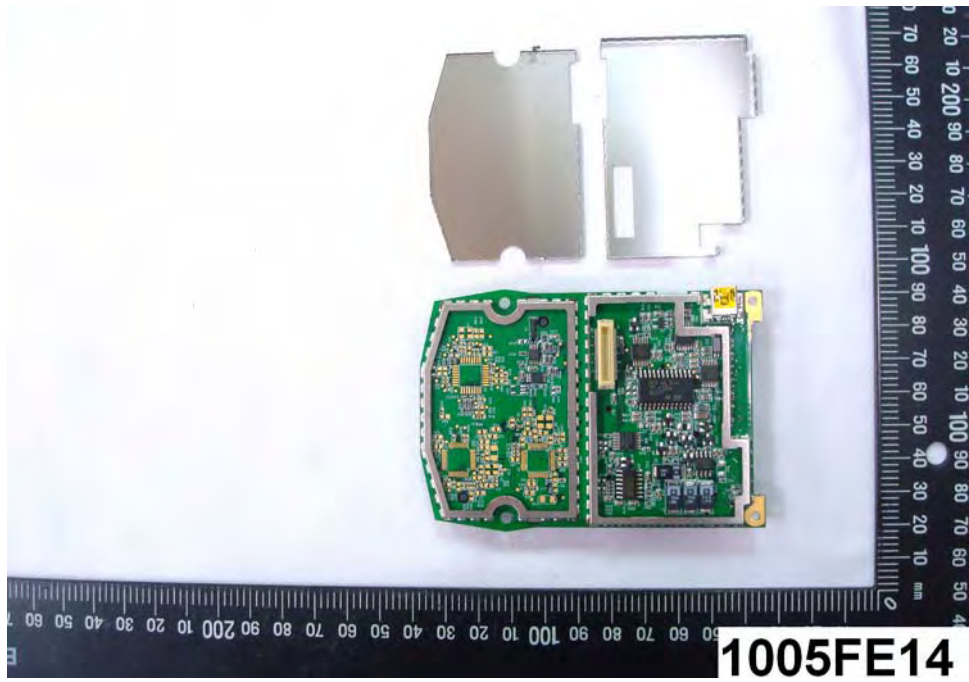
(19) EUT Photo
