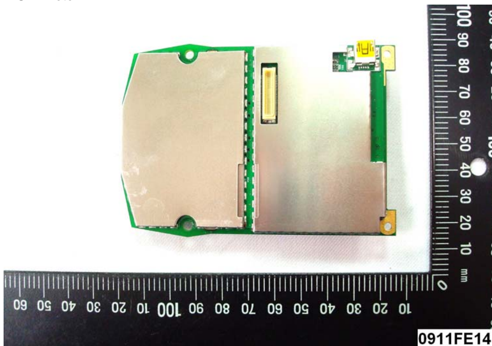
(18) EUT Photo
