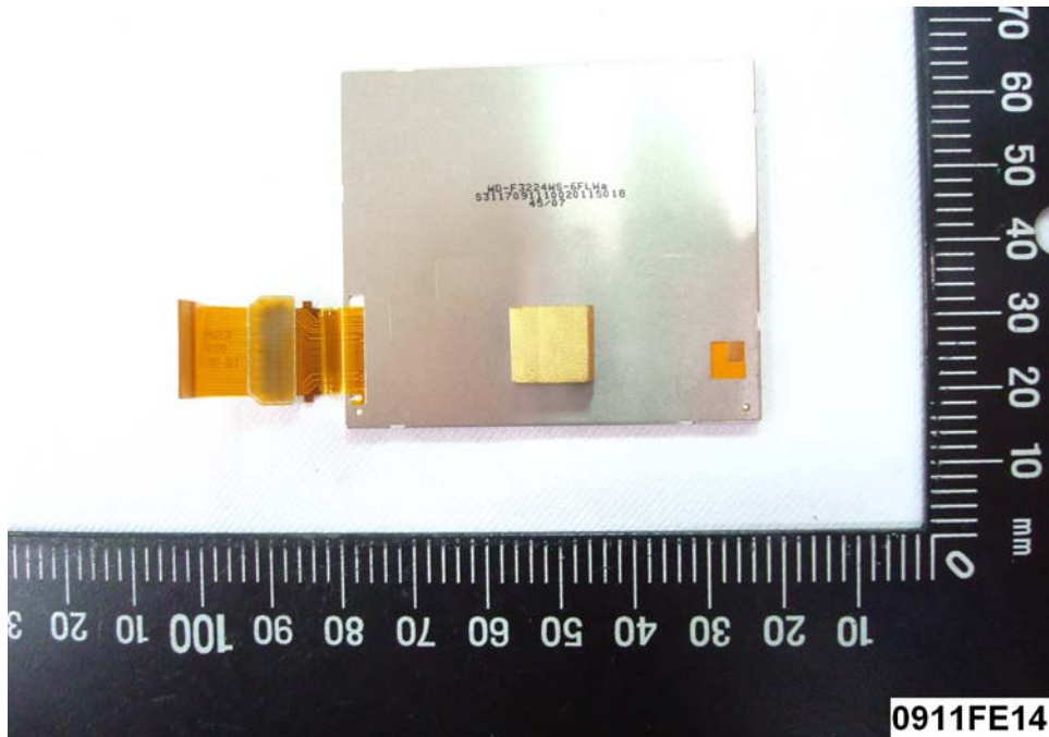
(31) EUT Photo
