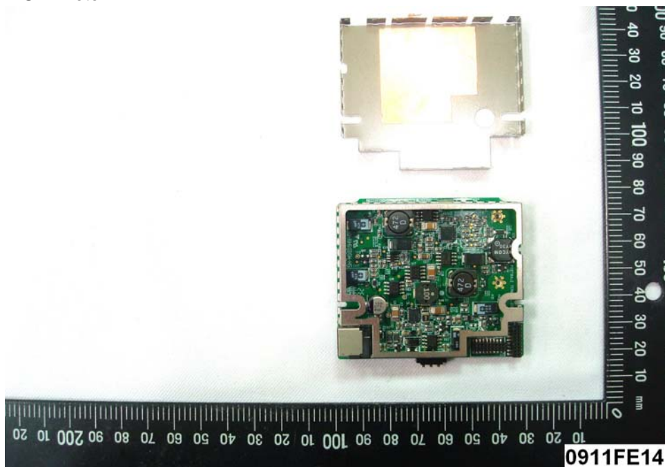
(14) EUT Photo
