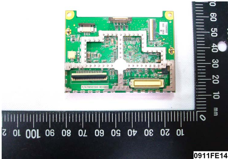
(24) EUT Photo
