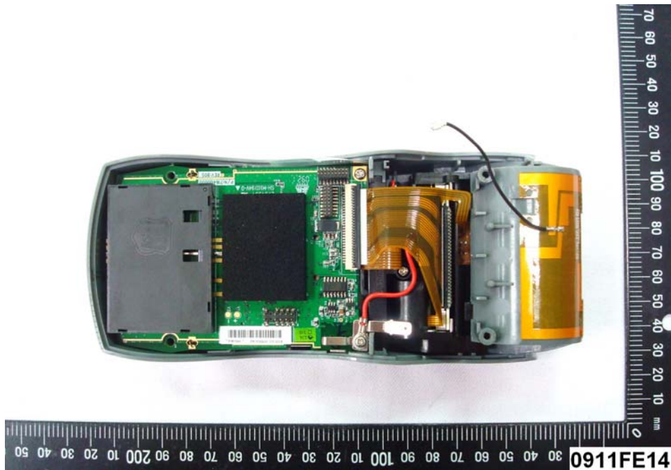
(16) EUT Photo
