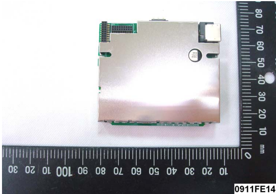
(13) EUT Photo
