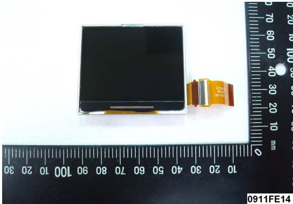
(30) EUT Photo
