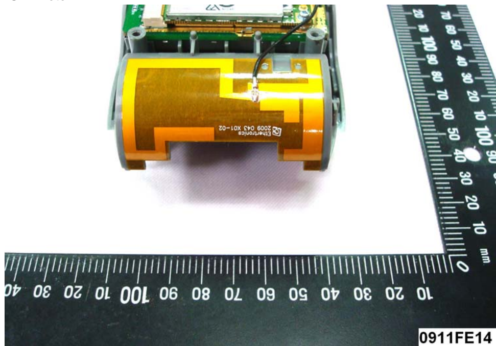
(6) EUT Photo
