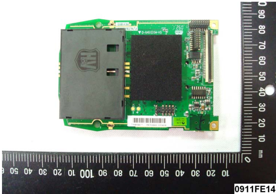
(17) EUT Photo
