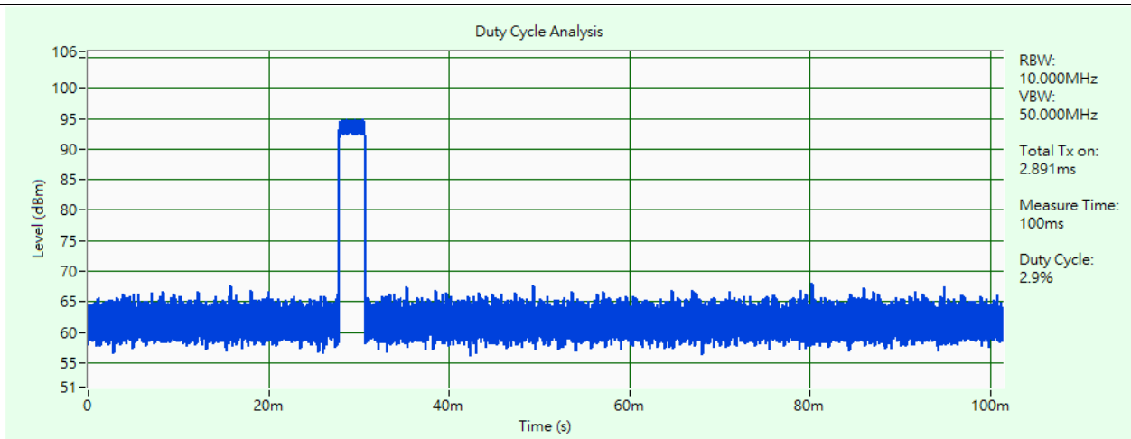
GFSK
