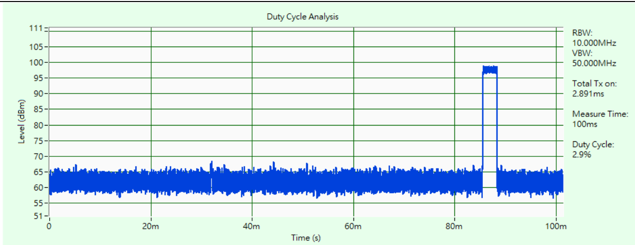
8DPSK
