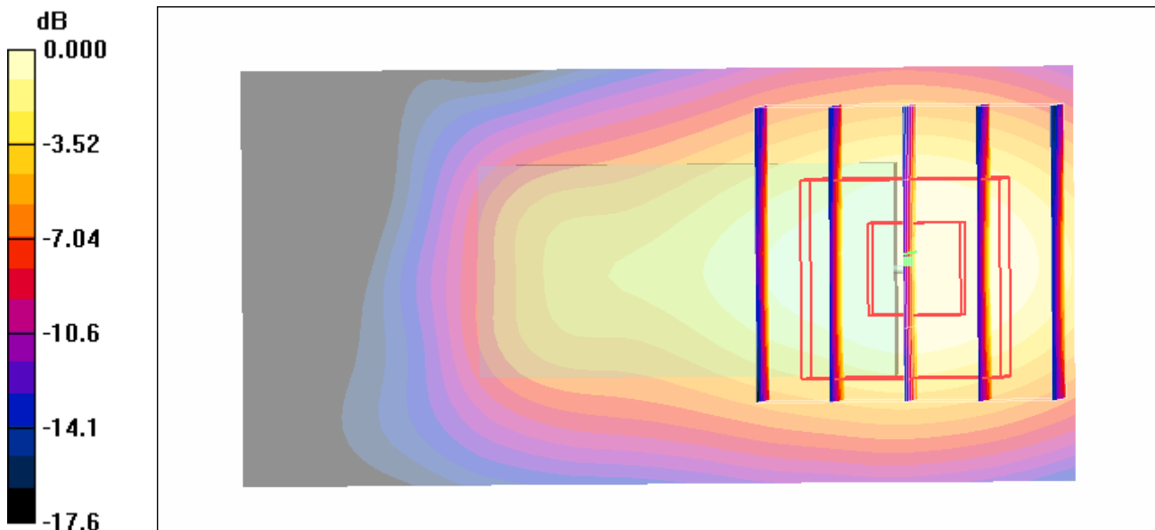
0 dB = 0.148mW/g
