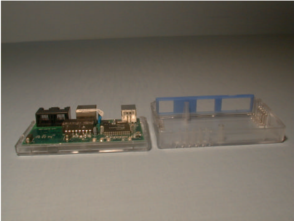
(4) EUT Photo
