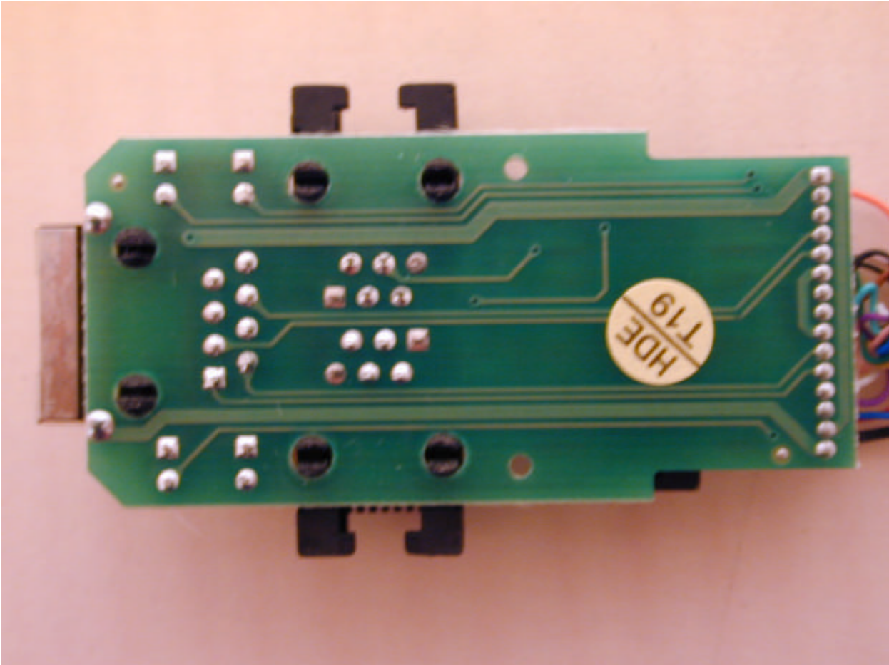
(12) EUT Photo
