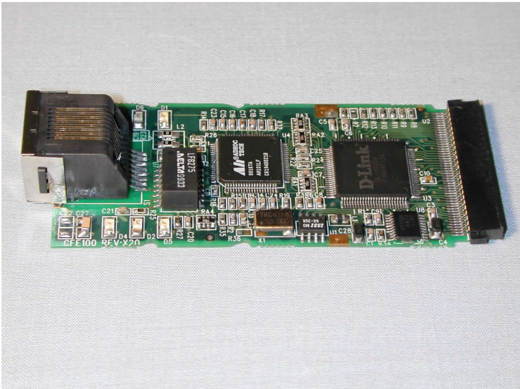
(6) EUT Photo
