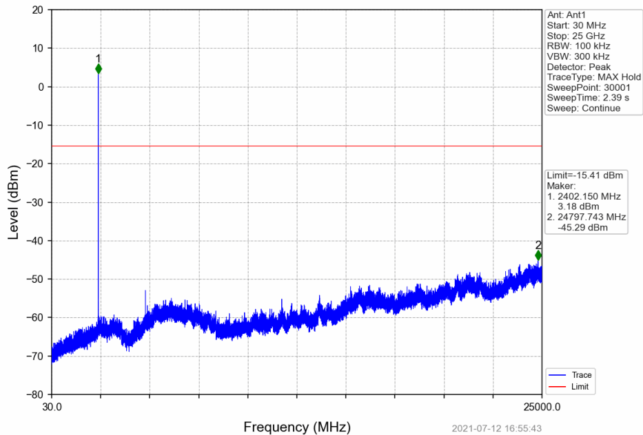
BLE 1M_LCH_2402MHz_DataRate=_Ant1_NTNV
