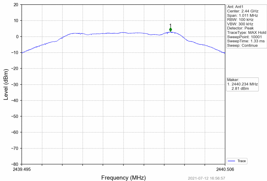
BLE 1M_MCH_2440MHz_DataRate=_Ant1_NTNV
