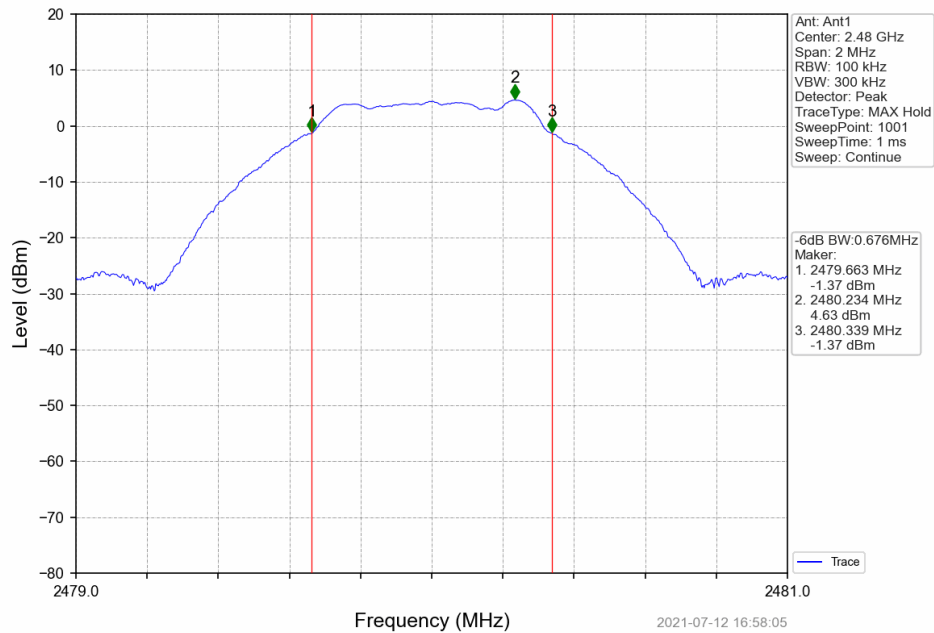
BLE 1M_HCH_2480MHz_DataRate=_Ant1_NTNV
