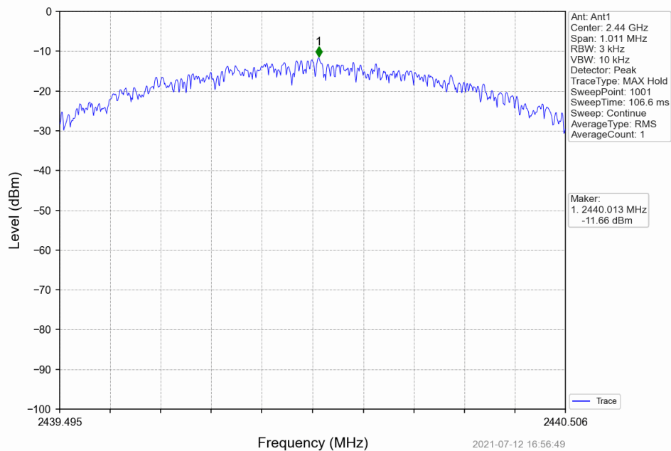
BLE 1M_MCH_2440MHz_DataRate=_Ant1_NTNV
