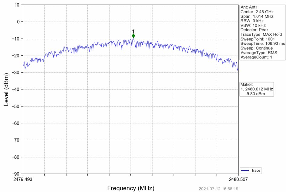
BLE 1M_HCH_2480MHz_DataRate=_Ant1_NTNV
