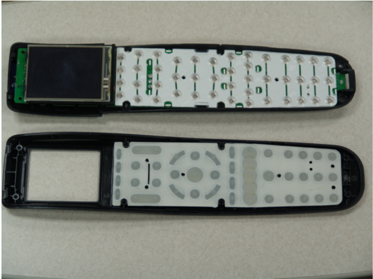
Top PCB
