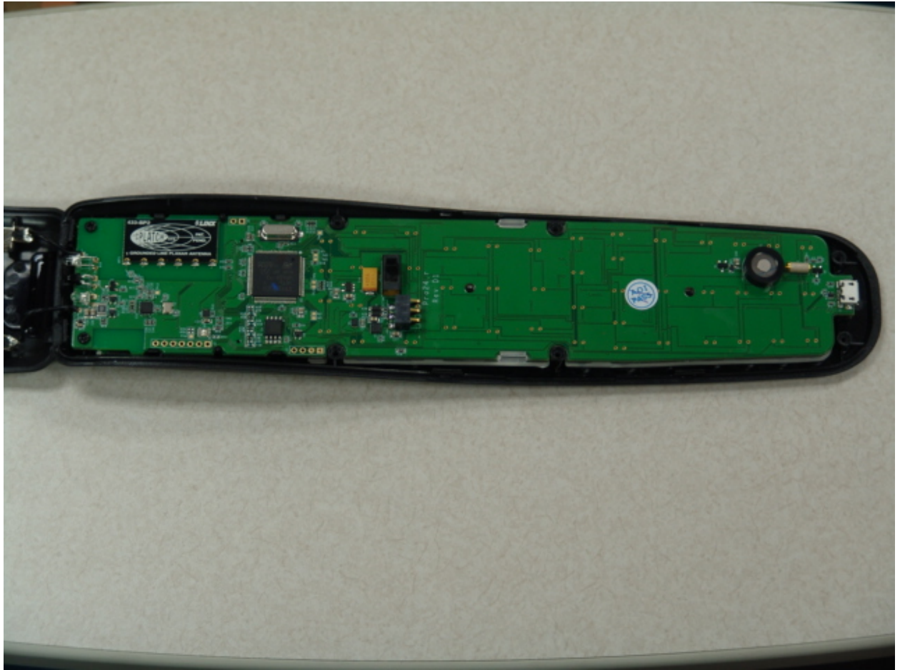
Bottom PCB
