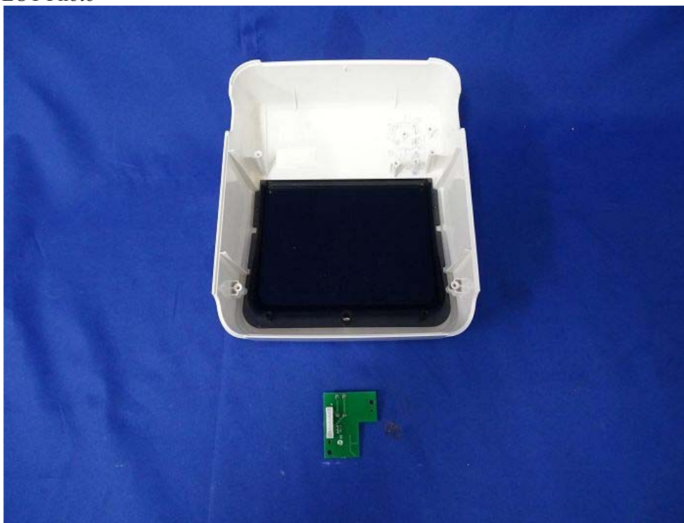
(30) EUT Photo
