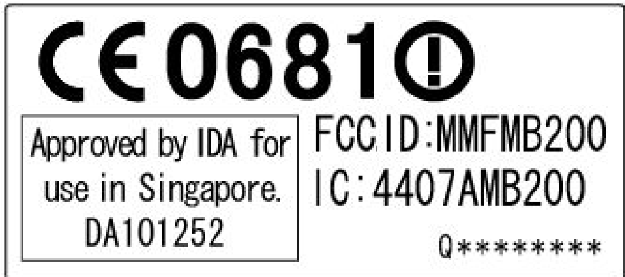
EUT Bottom Face
