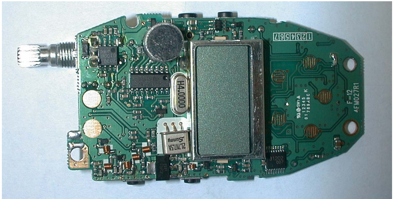
PCB Top
