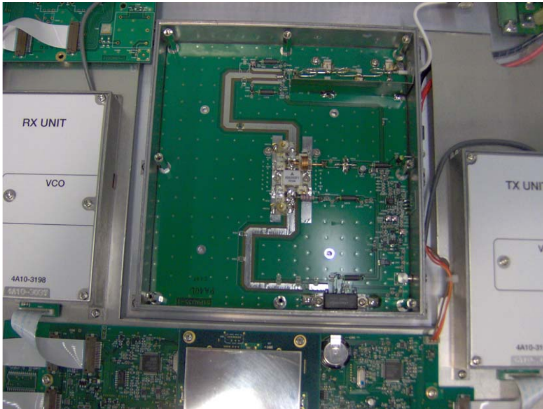
50 W PA TOP
