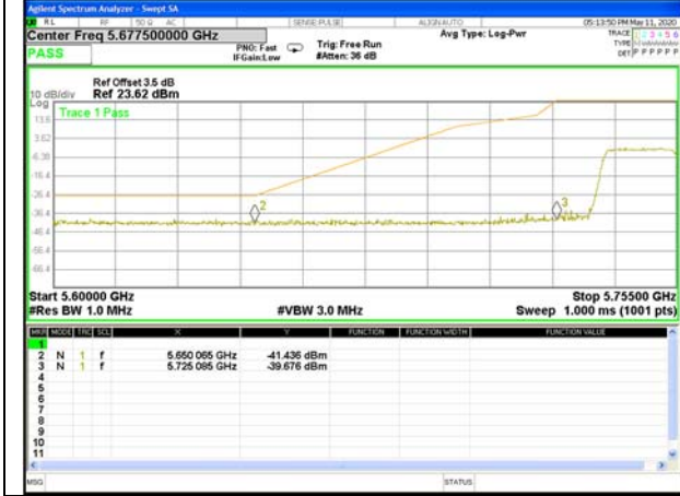
W58_11n40_Lower_Band edge
