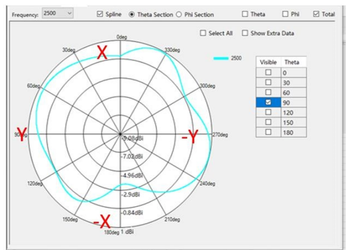
H面
