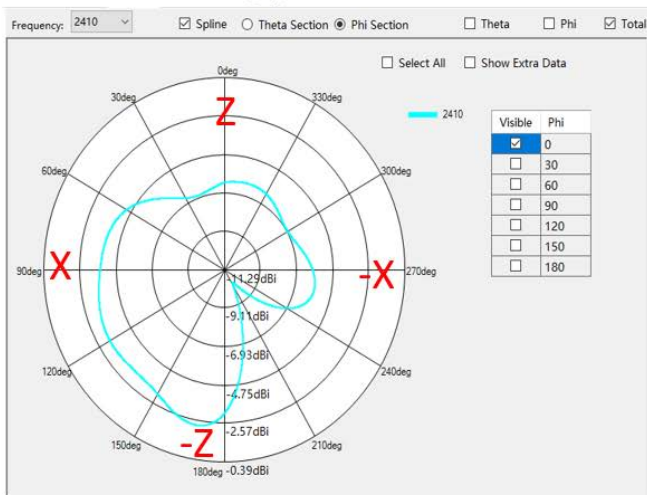
E1面
