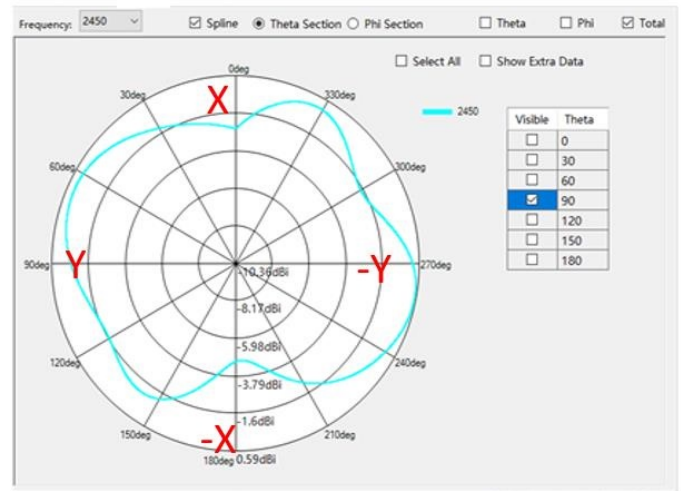
H面
