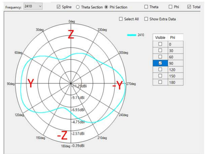
E2面
