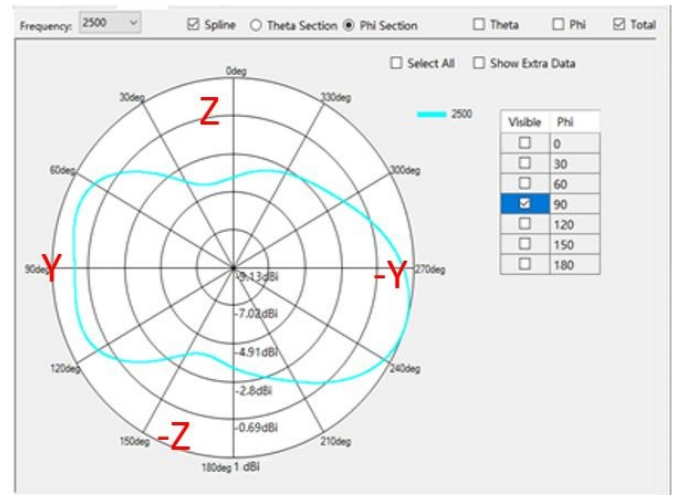
E2面
