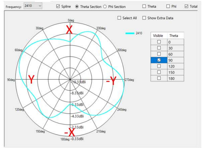
H面
