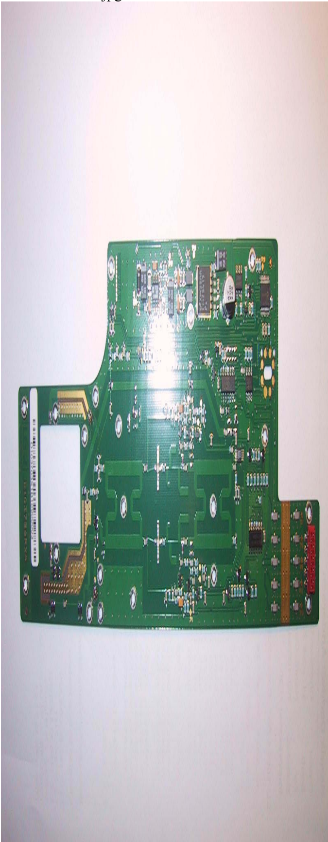
R2A-PCB TOP.jpg
