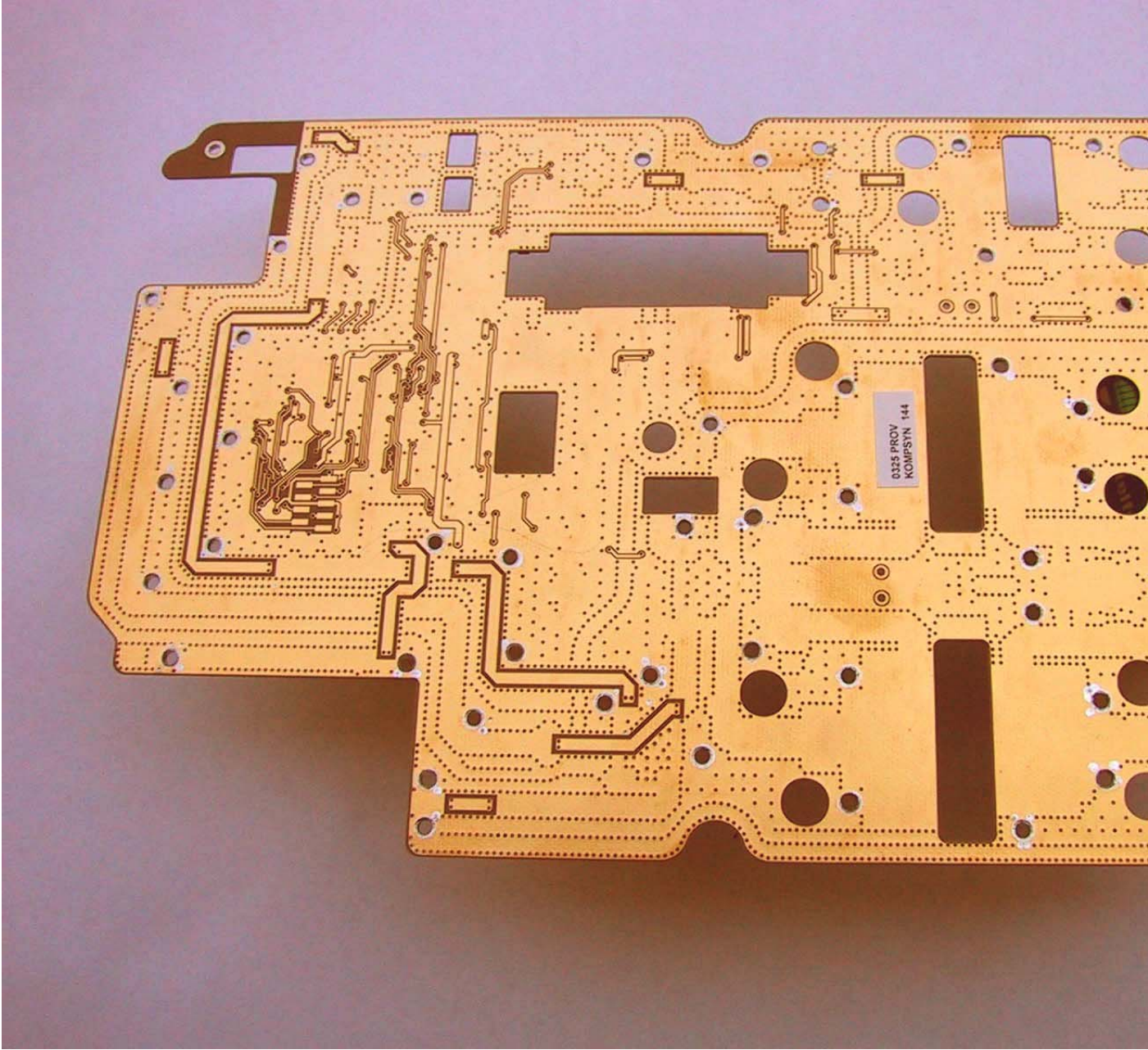
Back PA PCB.jpg
