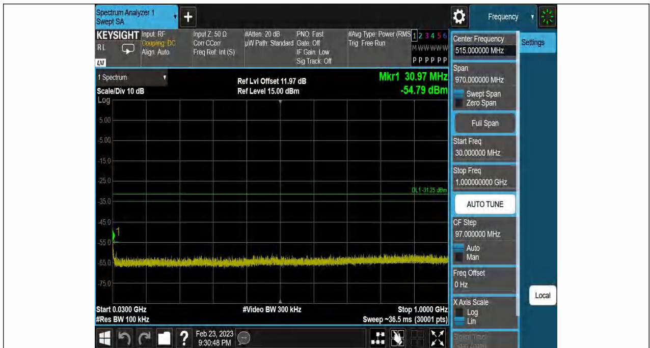
11N40SISO-Ant1-2452-30~1000--1.25
