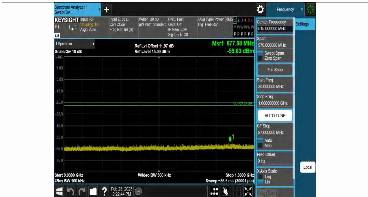
11G-Ant1-2462-30~1000-2.45
