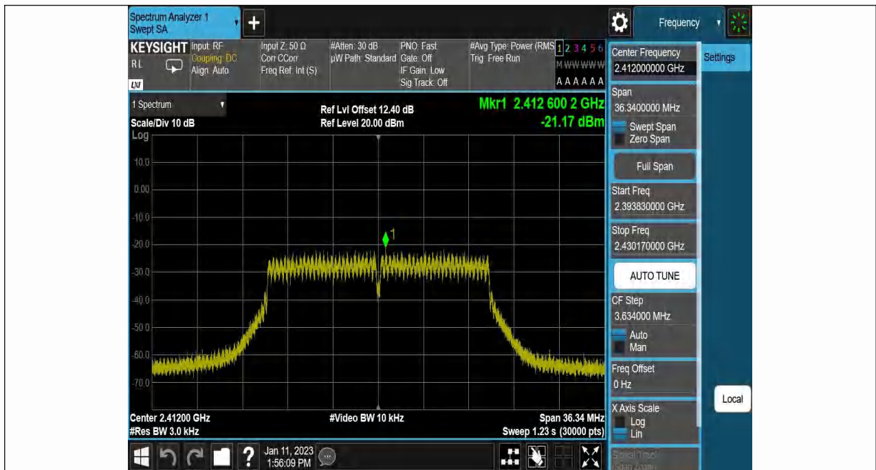
11N20SISO-Ant1-2412--21.45-0.28-0.00-0.00
