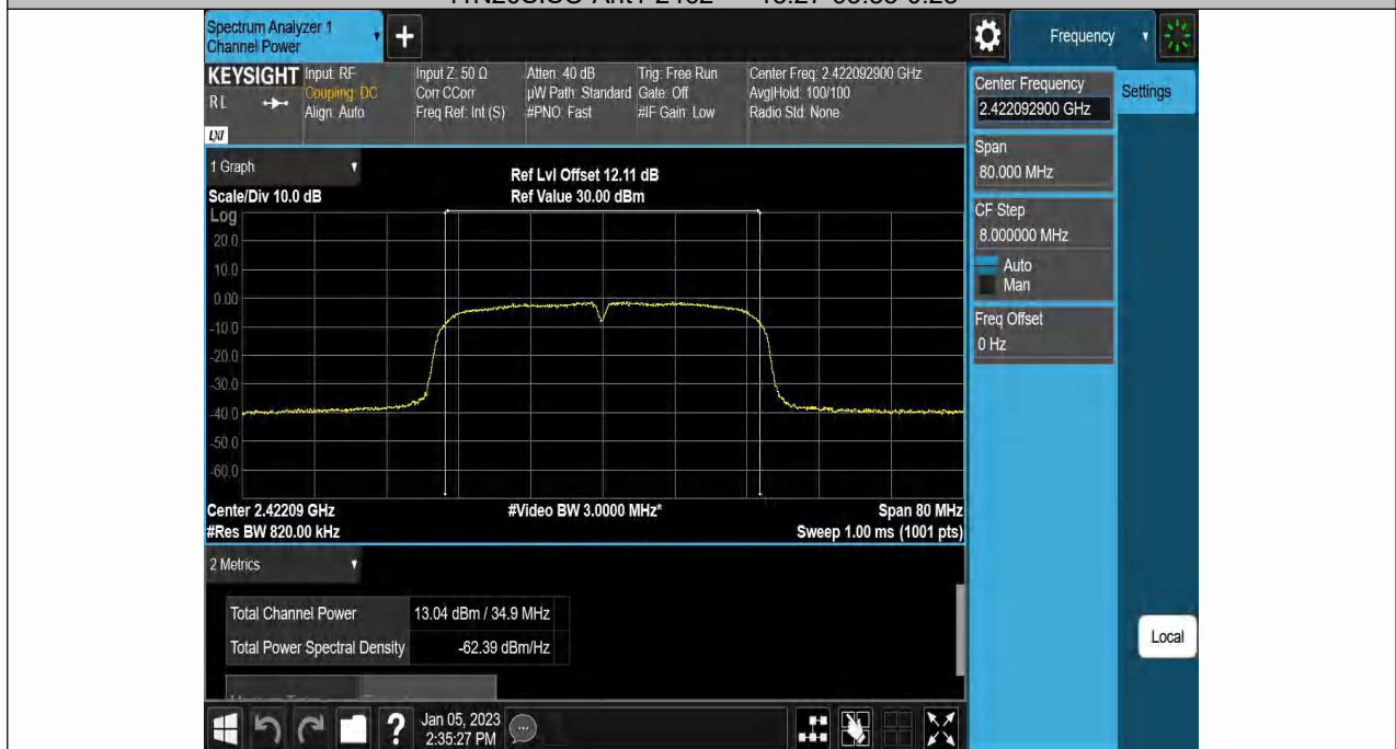
11N40SISO-Ant1-2422-----12.99-98.80-0.05
