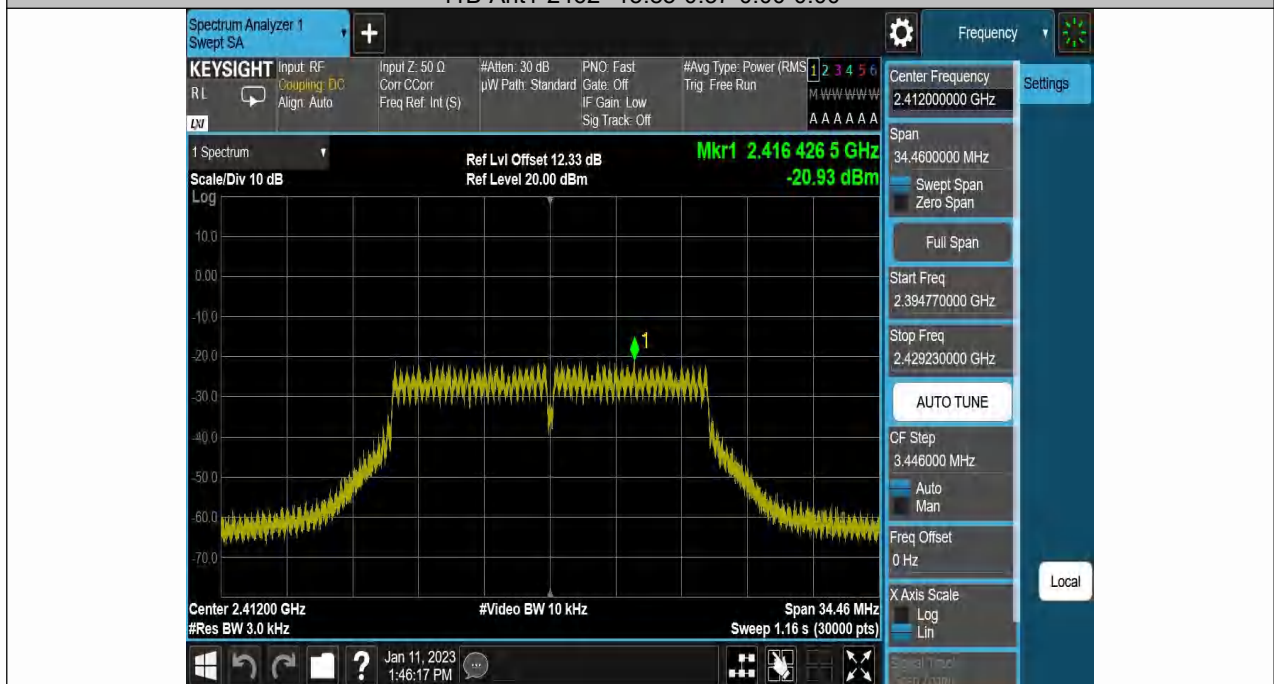
11G-Ant1-2412--21.14-0.21-0.00-0.00
