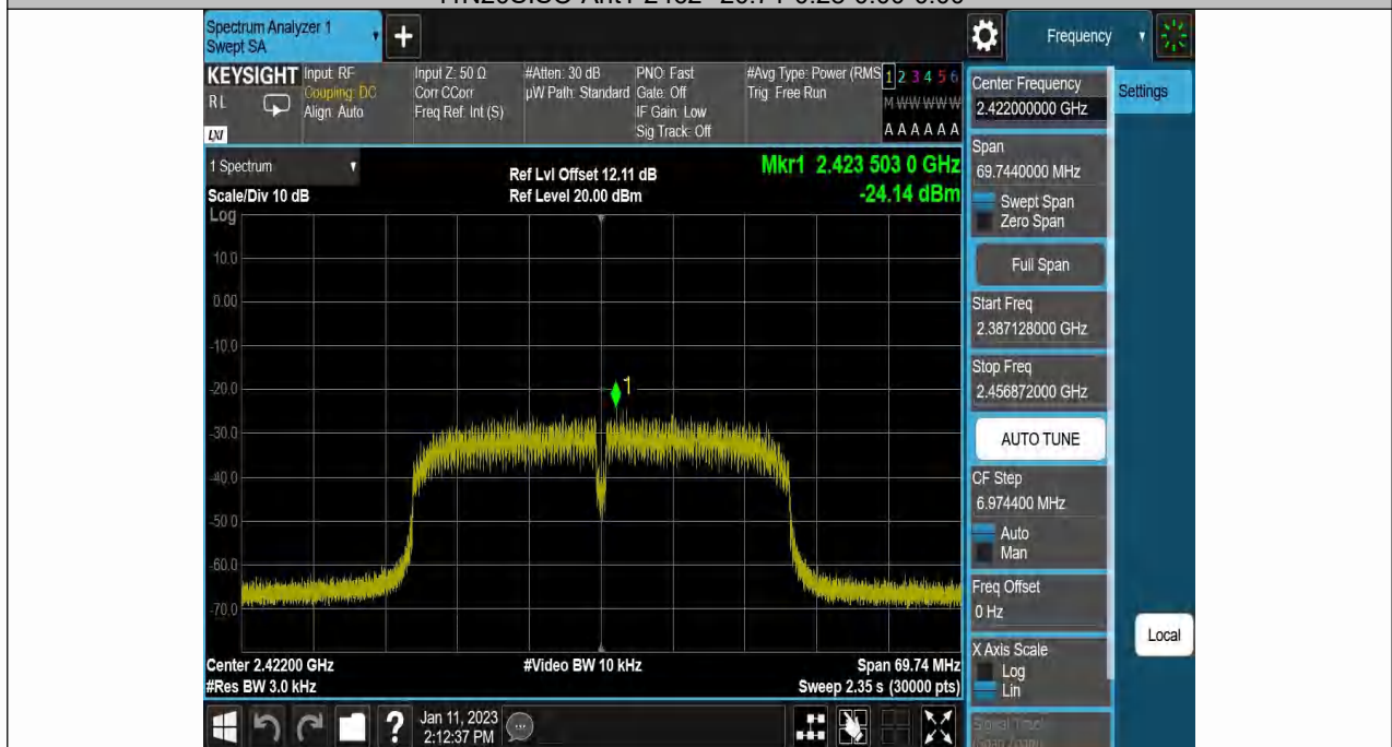
11N40SISO-Ant1-2422--24.19-0.05-0.00-0.00
