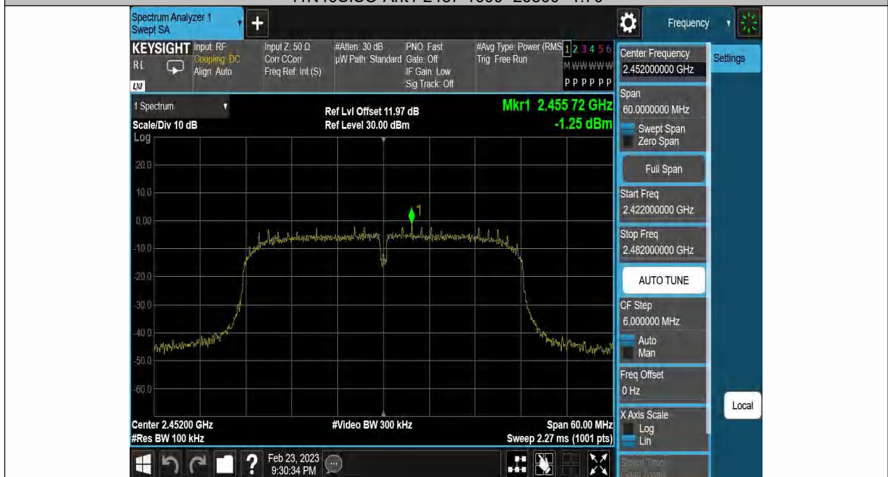
11N40SISO-Ant1-2452-0~Reference--1.25
