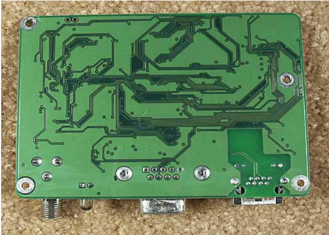
PCB 2 Bottom
