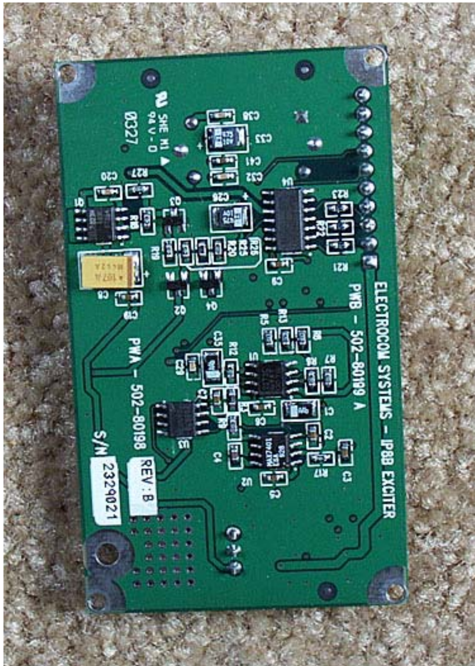
PCB 4 Bottom
