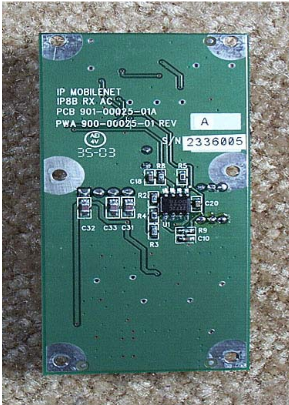
PCB 1 Bottom
