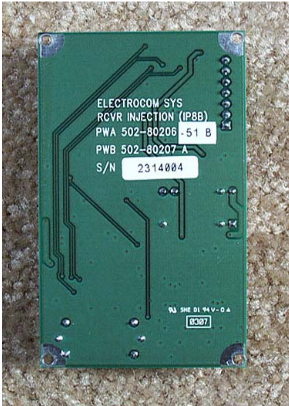
PCB 2 Bottom
