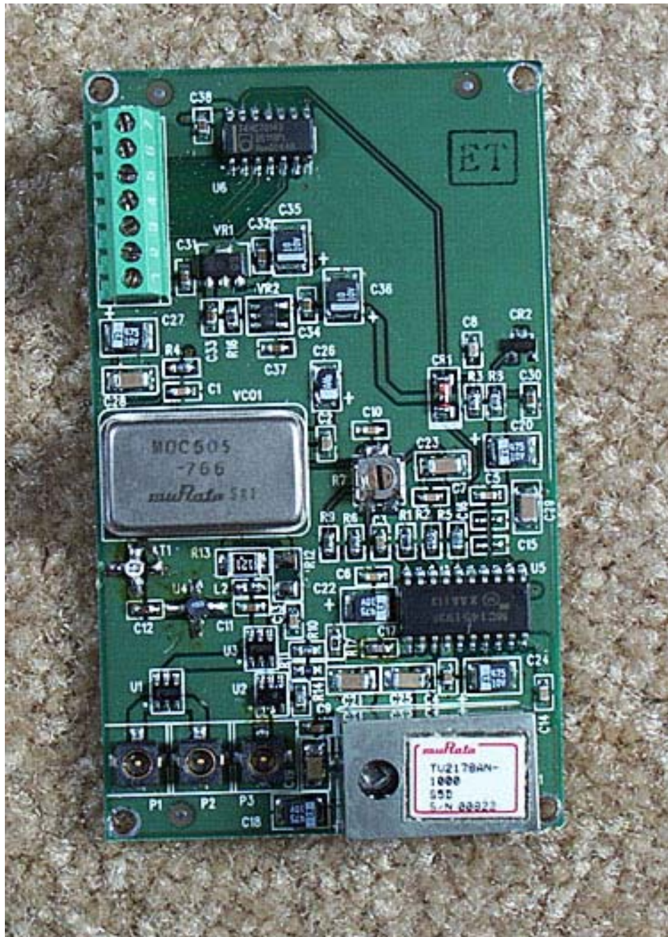
PCB 2 Top
