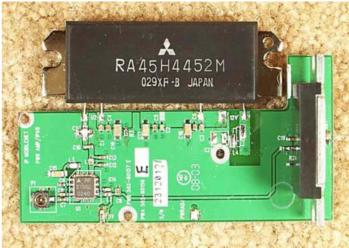
PCB TX Output Top
