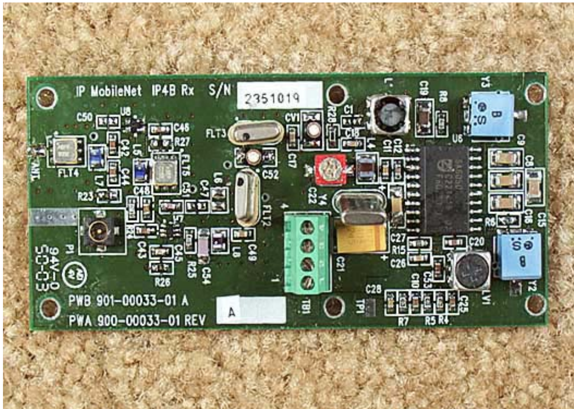
PCB RX Top
